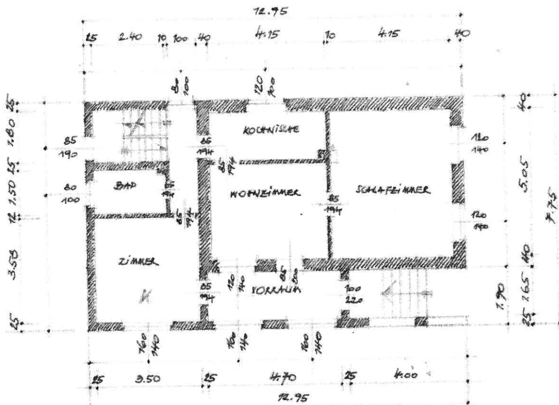
ERDGESCHOSS
