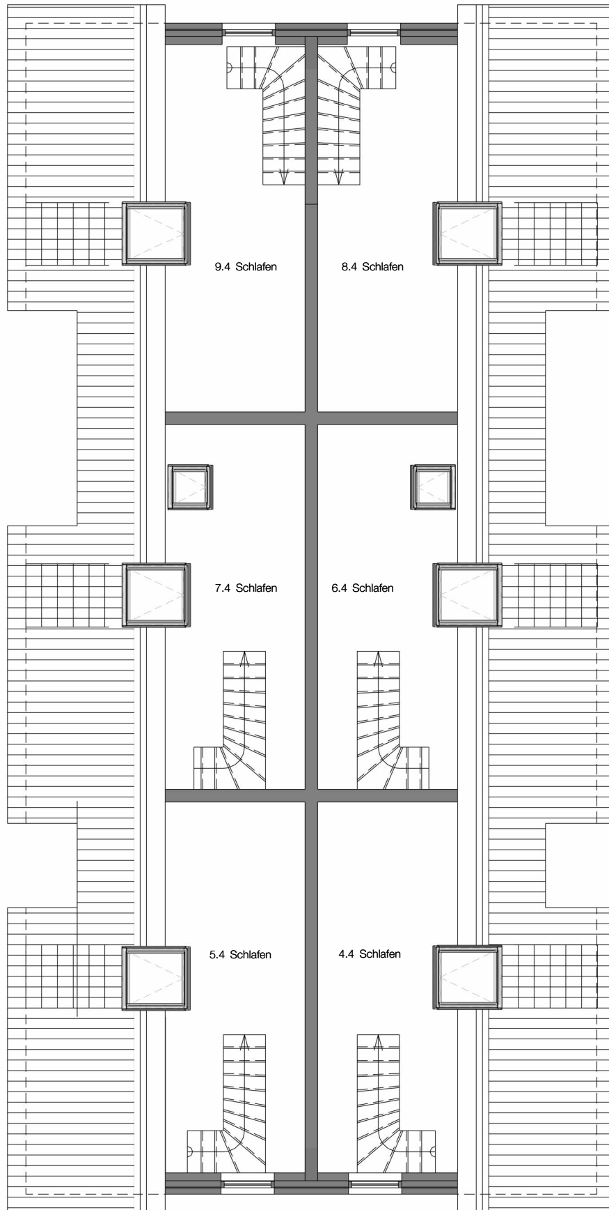
Dachgeschoss 2.Ebene M.1:100
