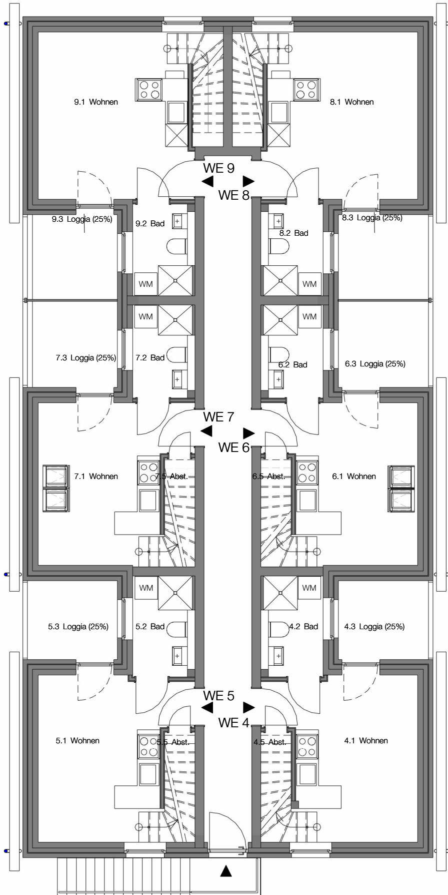
Dachgeschoss M.1:100
