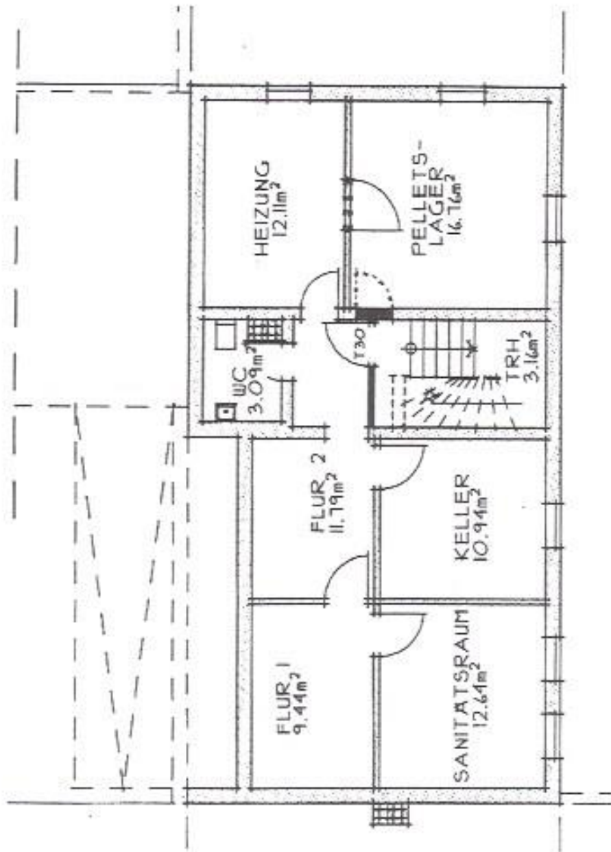
Kellergeschoss Bürogebäude
