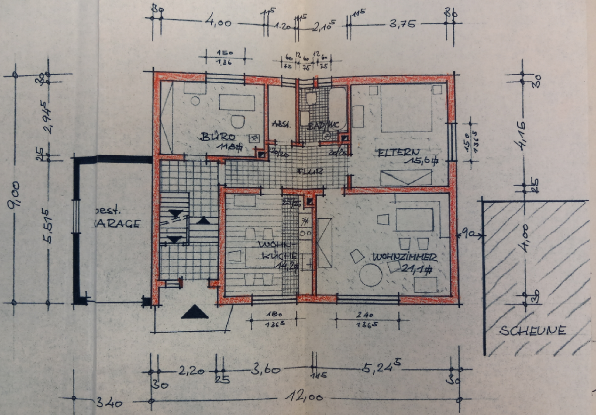
ERDGESCHOSSGRUNDRISS
