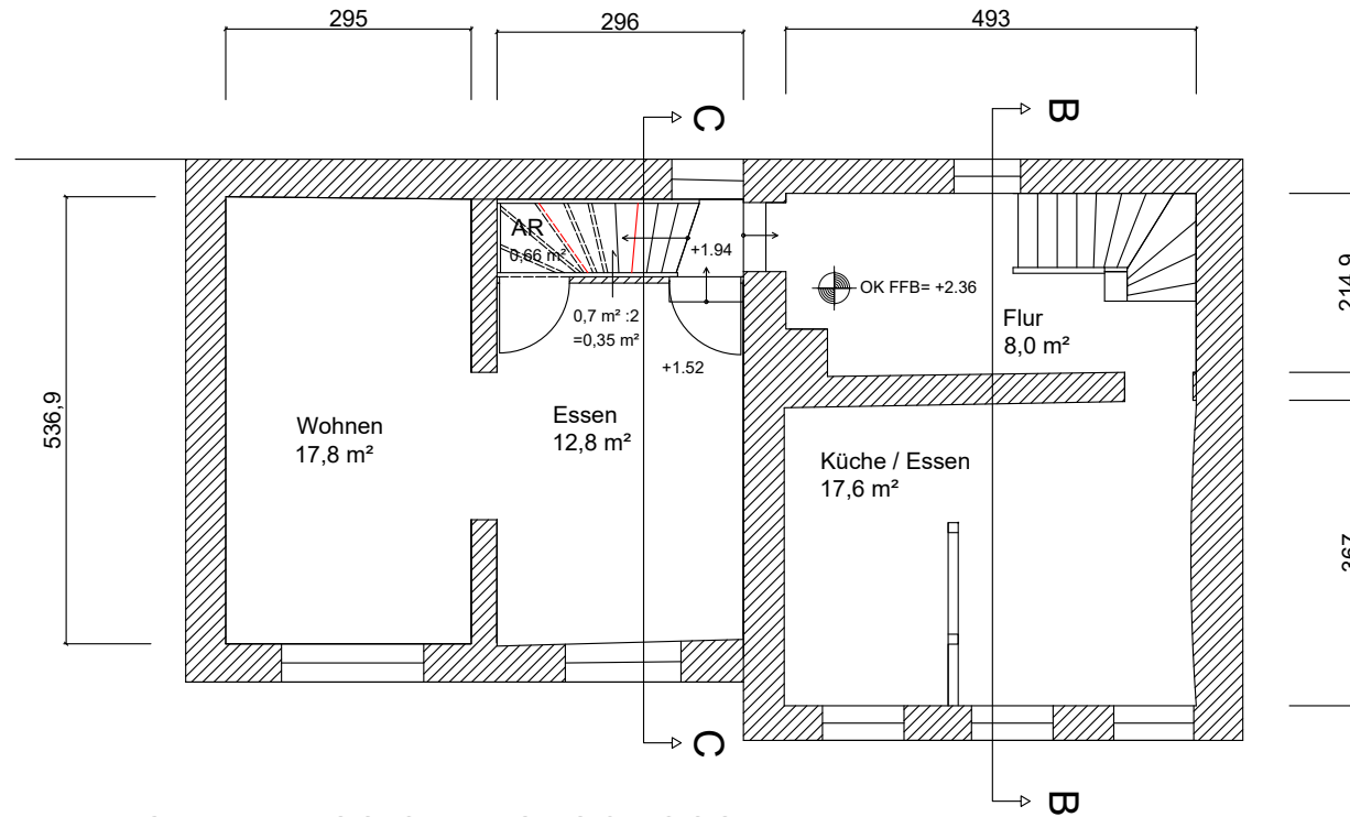
GRUNDRISS OBERGESCHOSS 1
