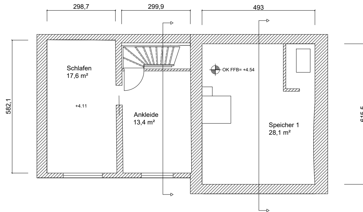
GRUNDRISS OBERGESCHOSS 2
