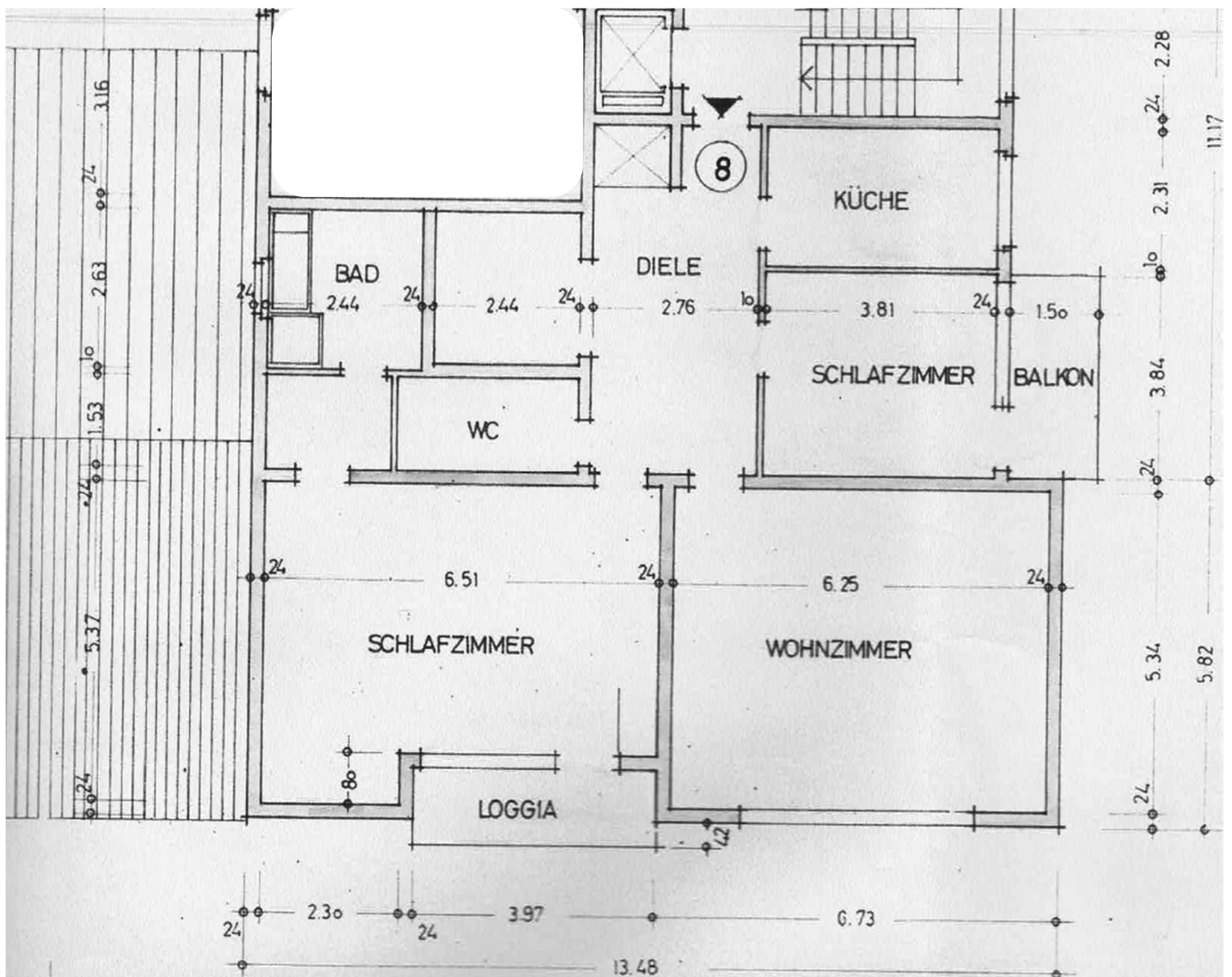
Grundriss Wohnung 8 in der zweiten Etage Graf-Recke-Str. 67 in 40239 Düsseldorf
