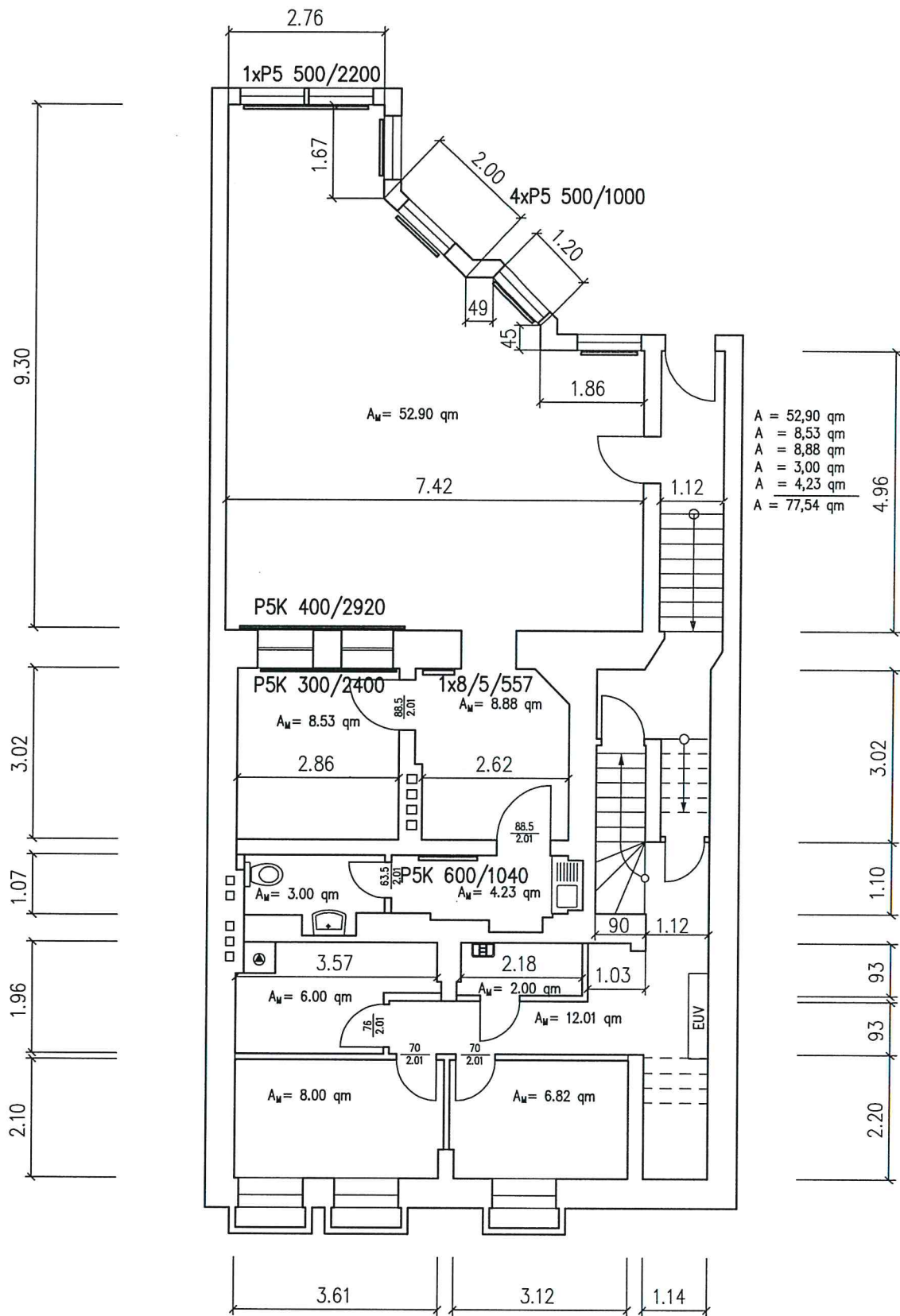
Kellergeschoß A_M \text{ gesamt} = 112.37 \text{ qm} M 1:100
