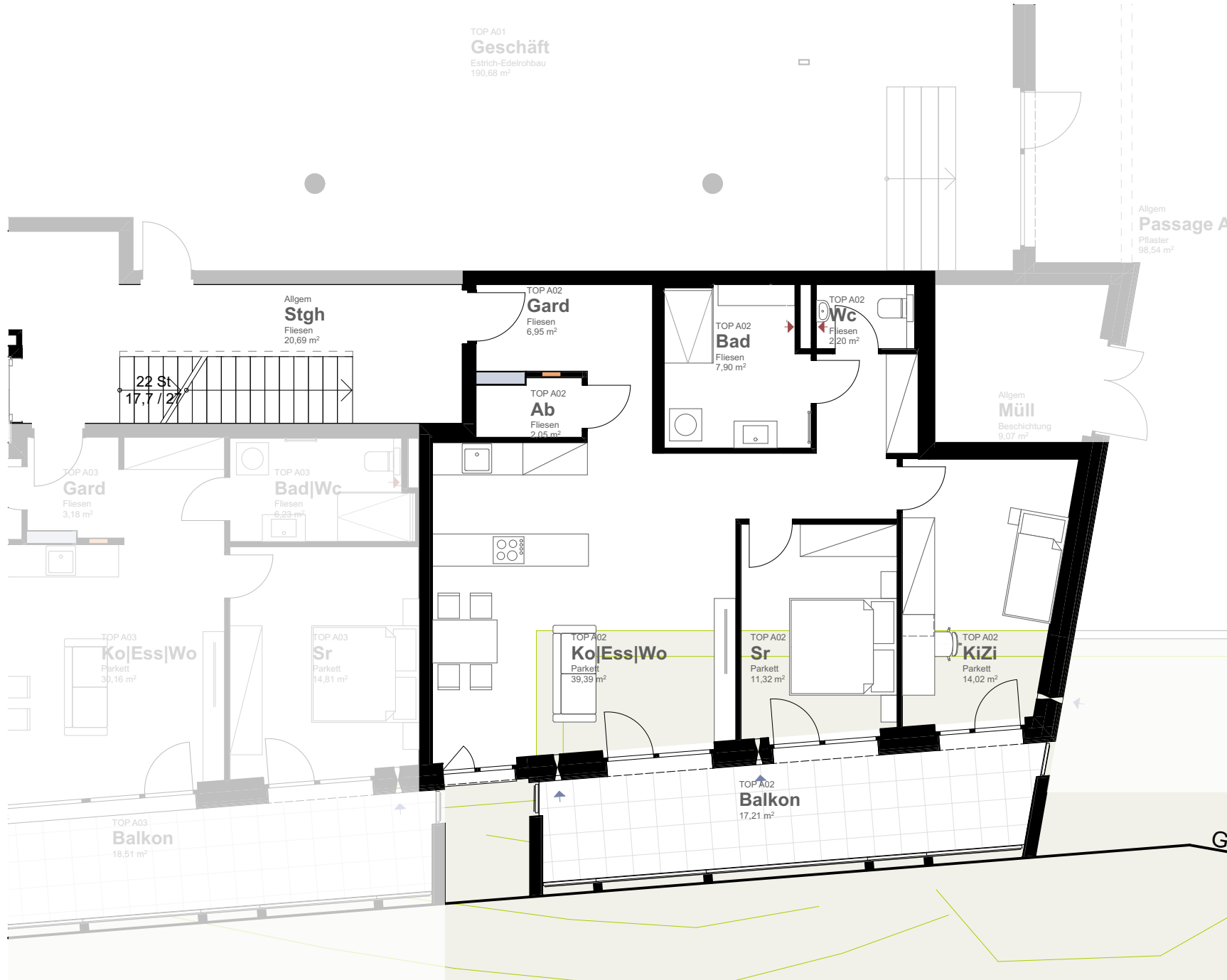
TopA02 - Haus A - EG
