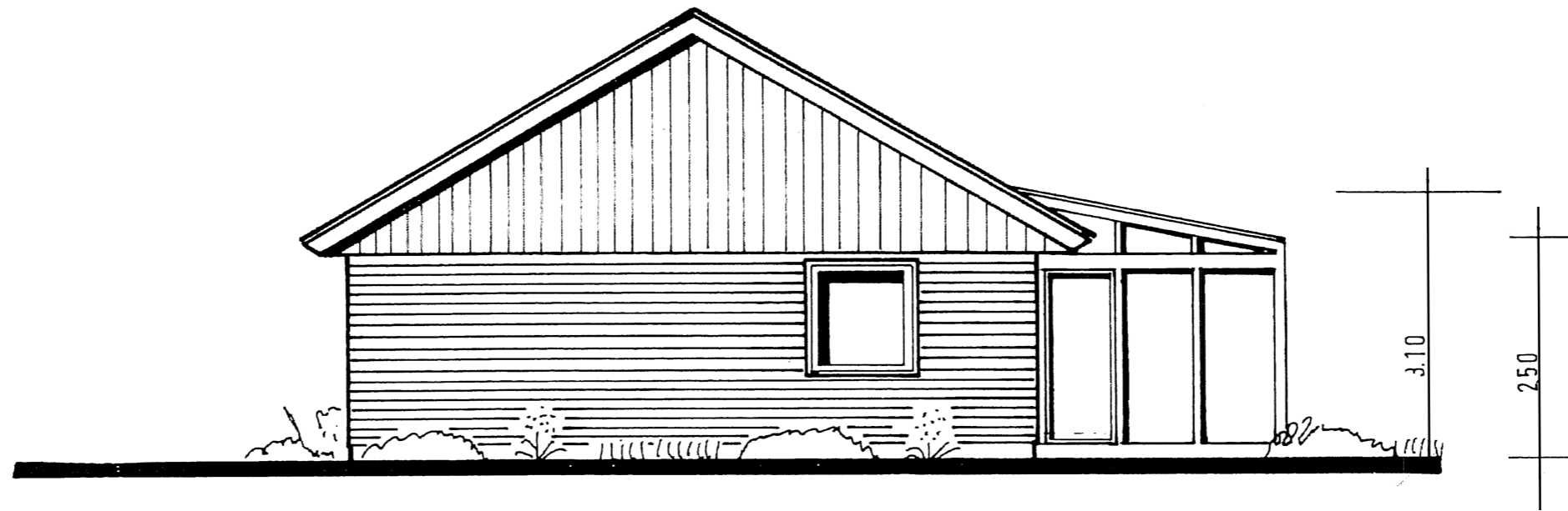
NORDANSICHT M-1:100
