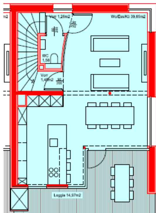
Grundriss EG M 1:100
