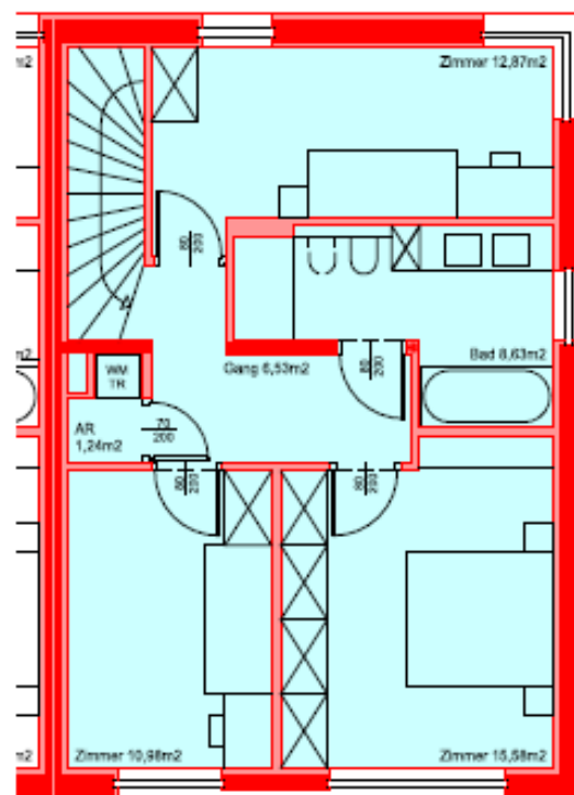
Grundriss OG M 1:100
