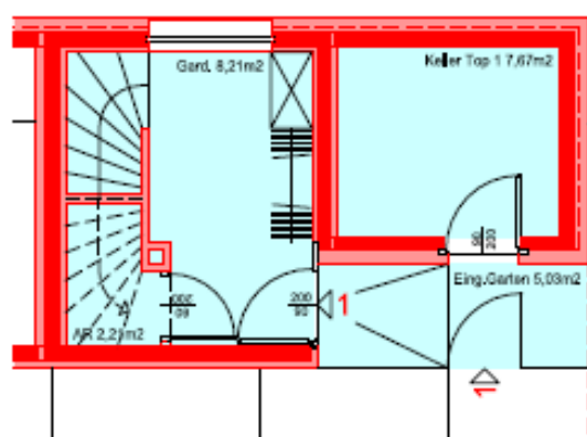
Grundriss UG M 1:100
