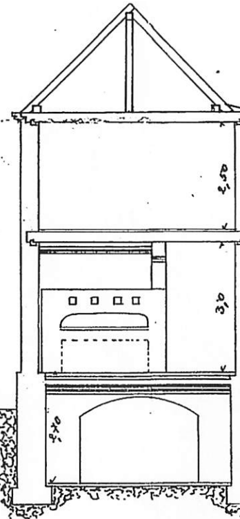
Schnitt A-B
