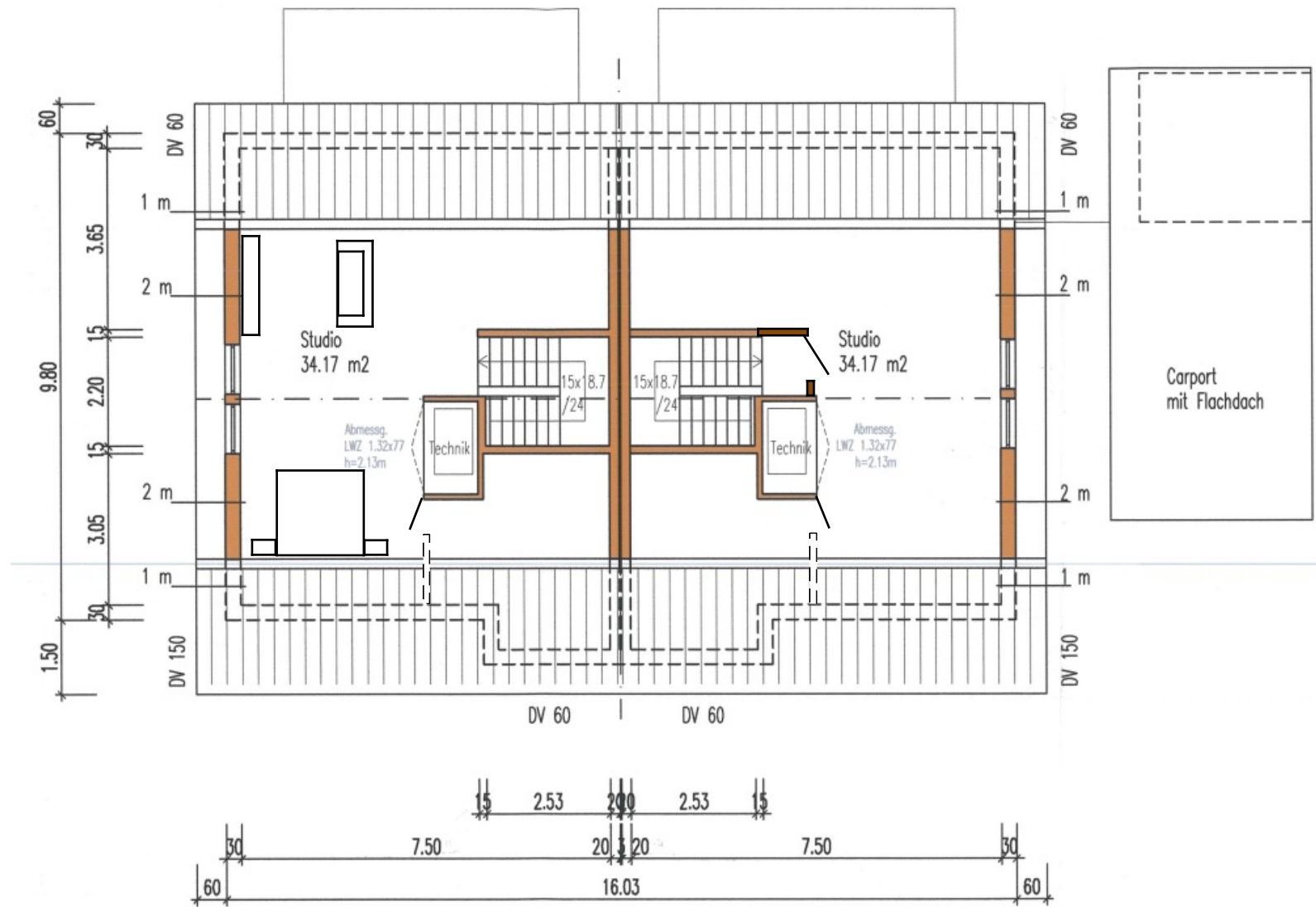
DACHGESCHOSS
