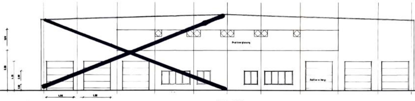
Ostansicht
