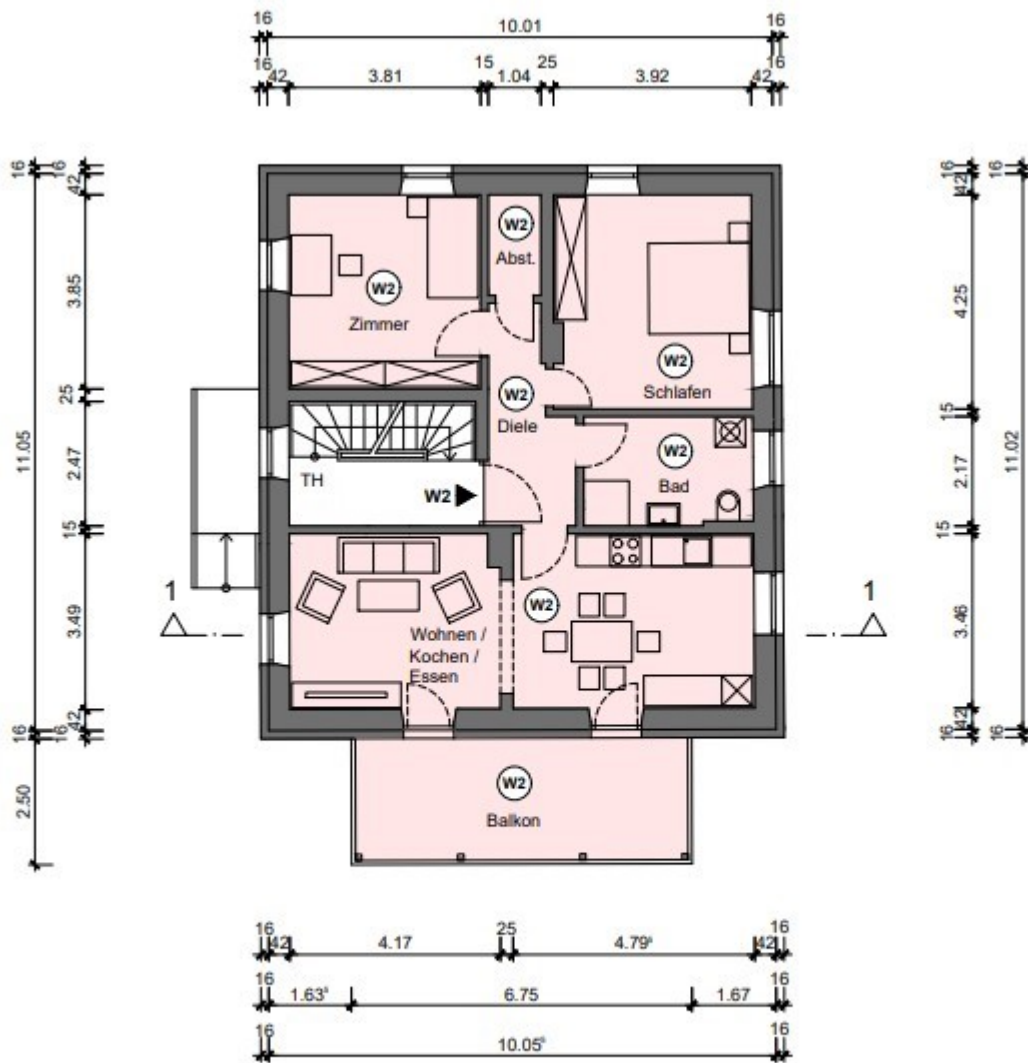
1. OBERGESCHOSS HAUPTGEBÄUDE
