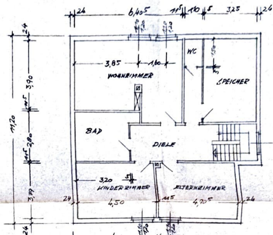
DACHGESCHOSS - AUGEBAUT
