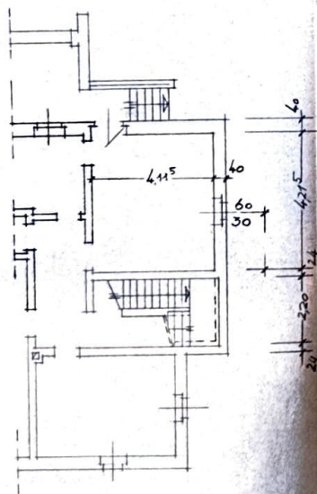
KELLERGECHOSS
