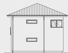
Ansicht Rechts
