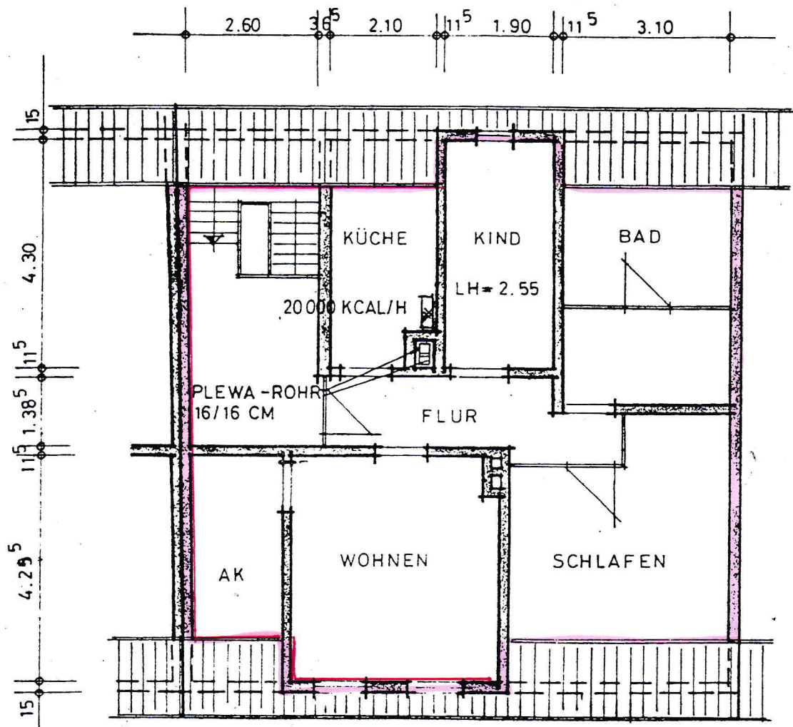
DACHGESCHOSS
