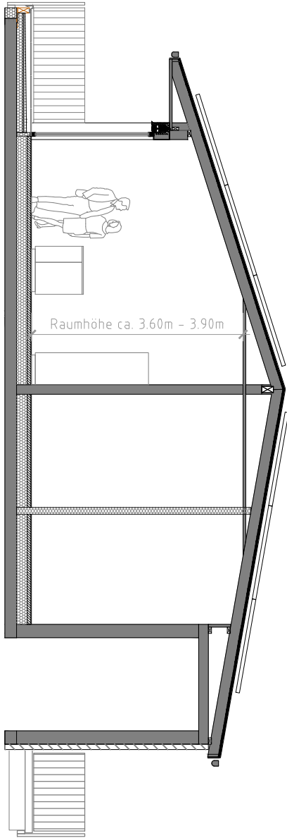
Schnitt A-A
