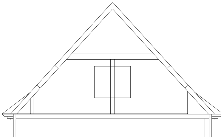
Schnitt A-A
