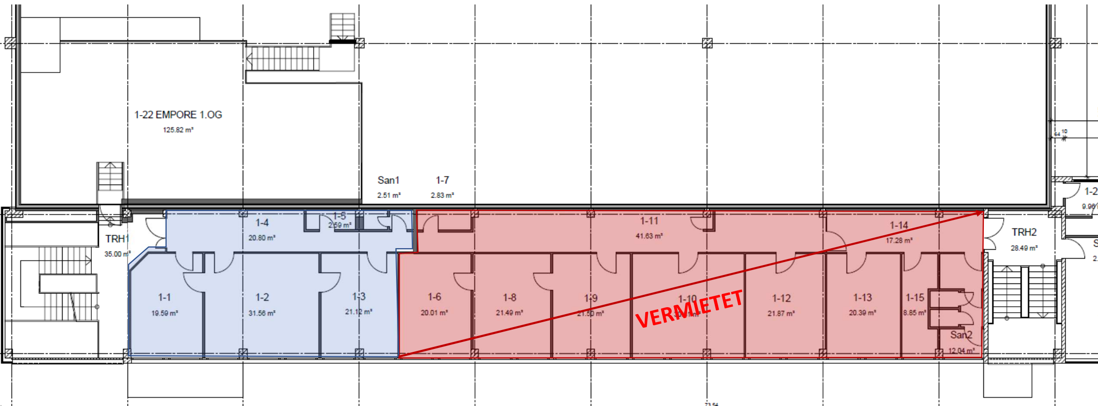
VH links – 1.OG mit ca. 107 qm
