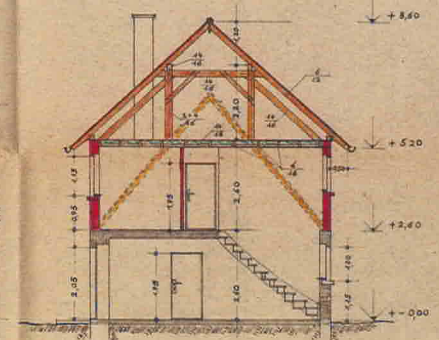
SCHNITT A-B
