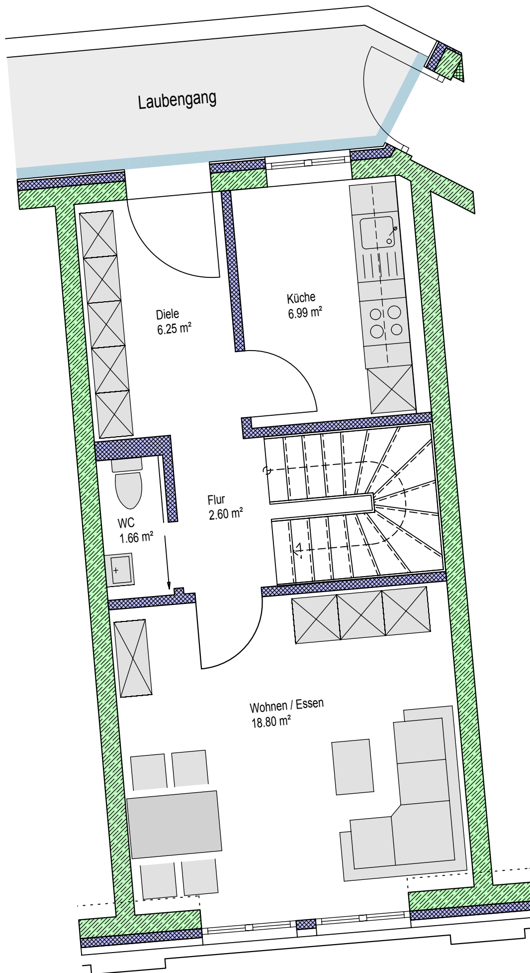
WOHNUNG 26 4.OBERGESCHOSS
