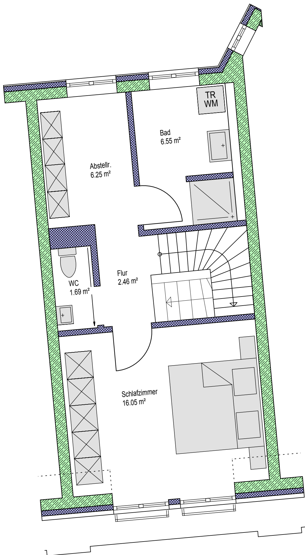
WOHNUNG 26 5.OBERGESCHOSS
