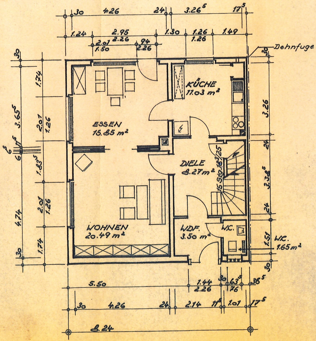
ERDGESCHOSS
