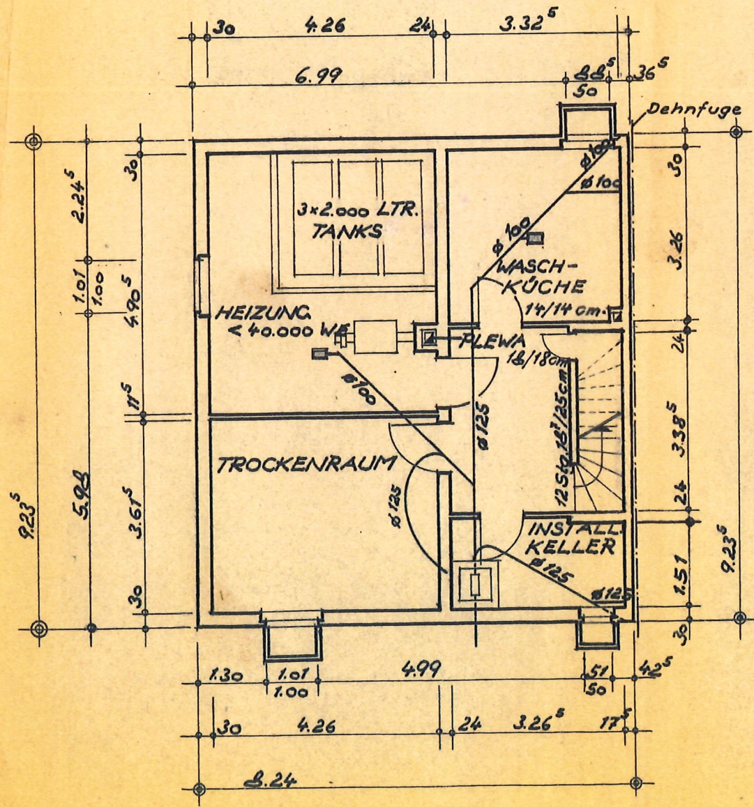
KELLERGEOSCHOSS
