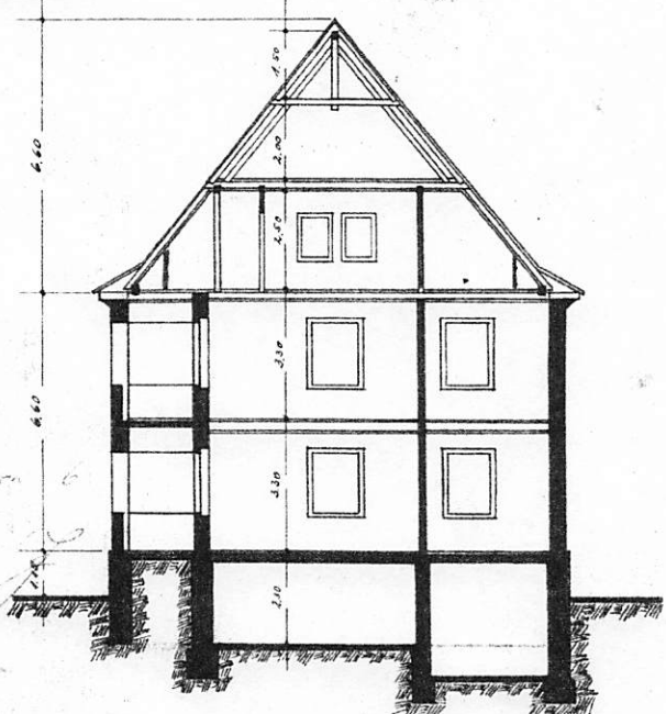
SEHNITT A-B.
