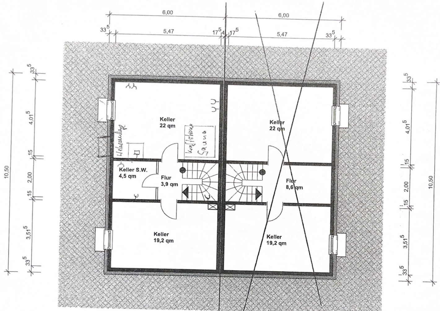
Exposé Typ A Kellergeschoss M 1:100 Datum: 27.11.18
