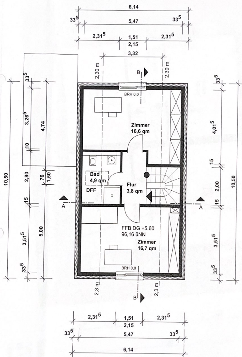
Dachgeschoss
