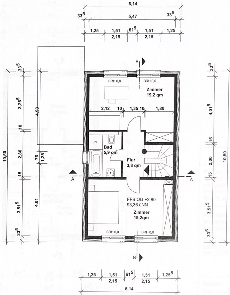
Obergeschoss
