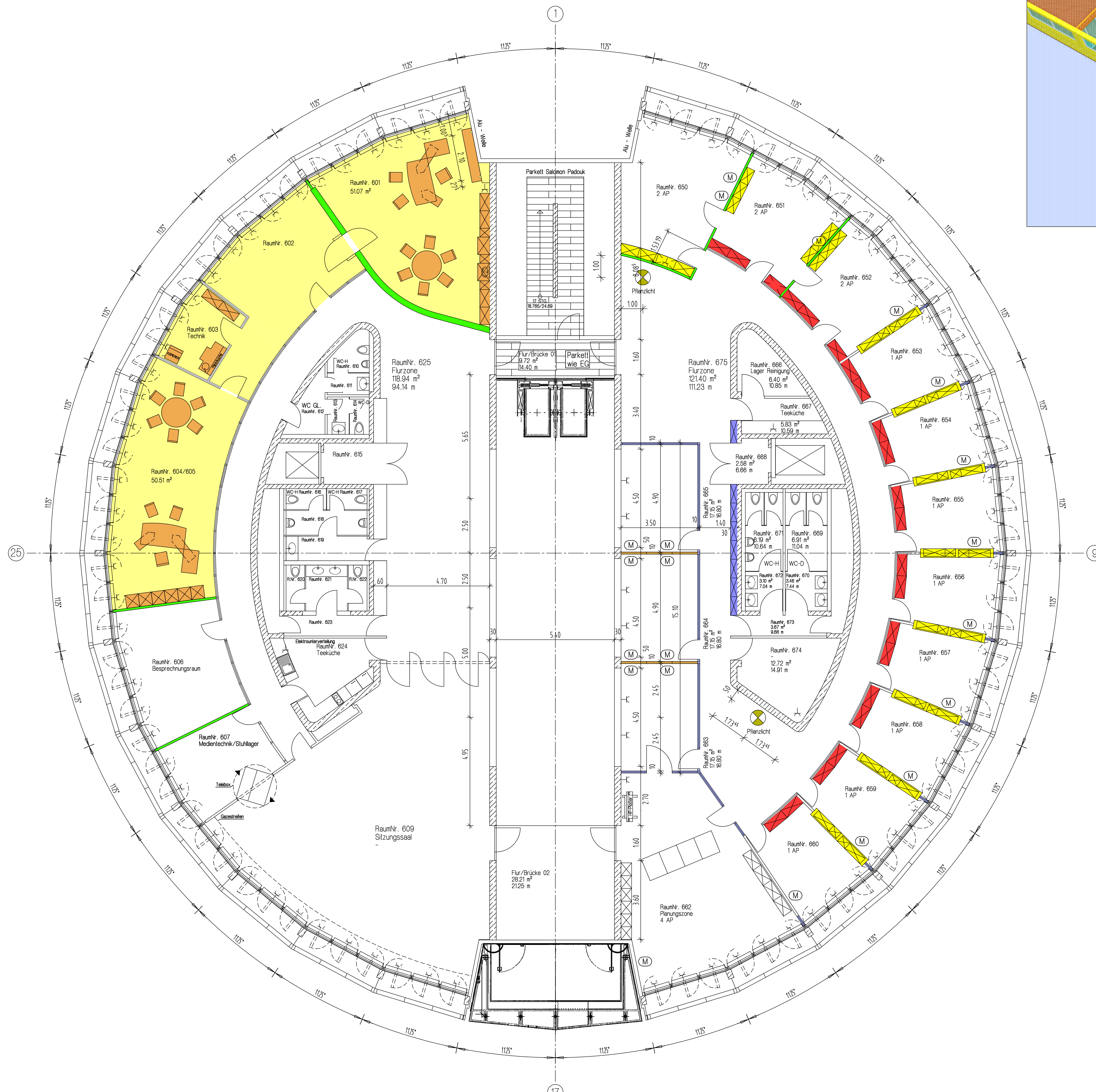
6. OBERGESCHOSS
