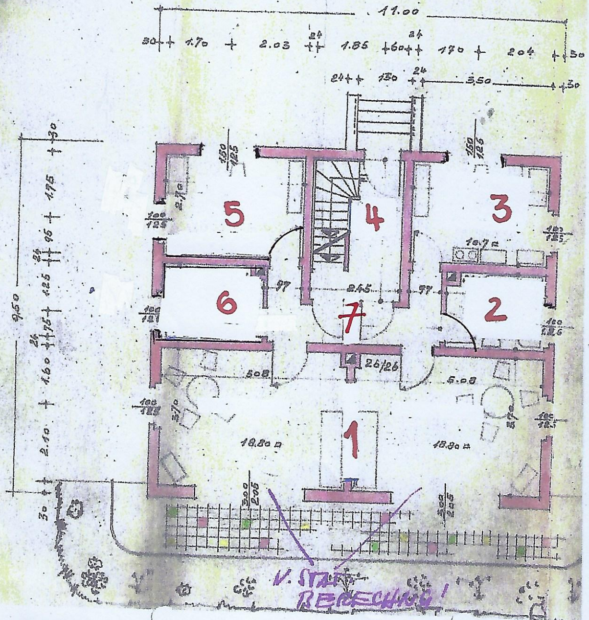
Geänderter Grundriß
