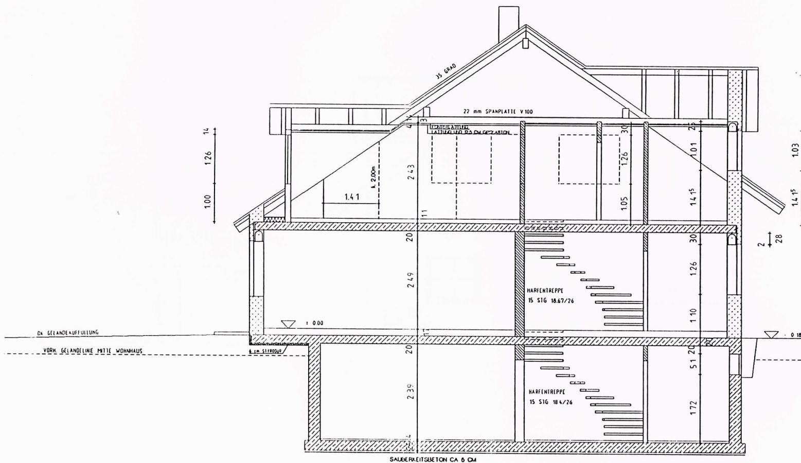
SCHNITT A-A
