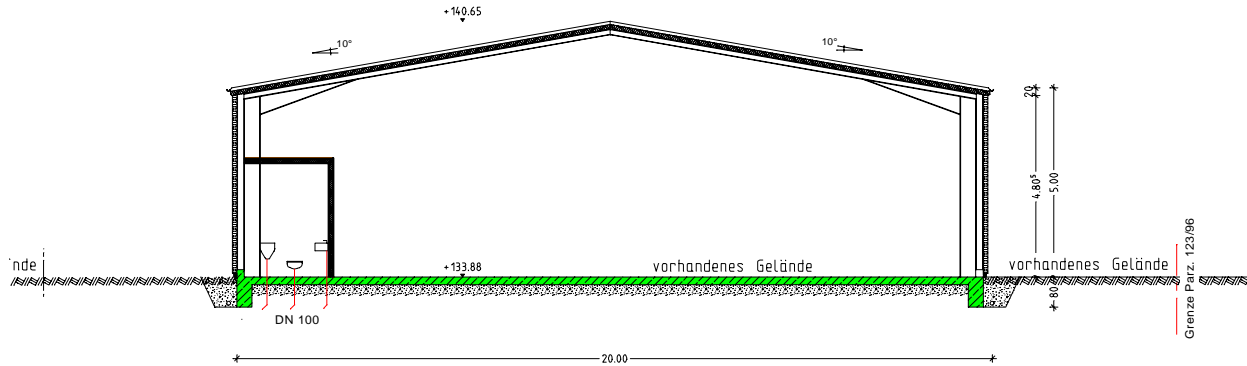
Schnitt B-B
