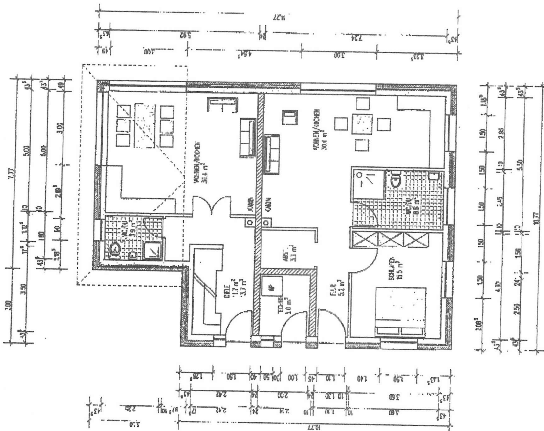
ERGUTSCHUSS
