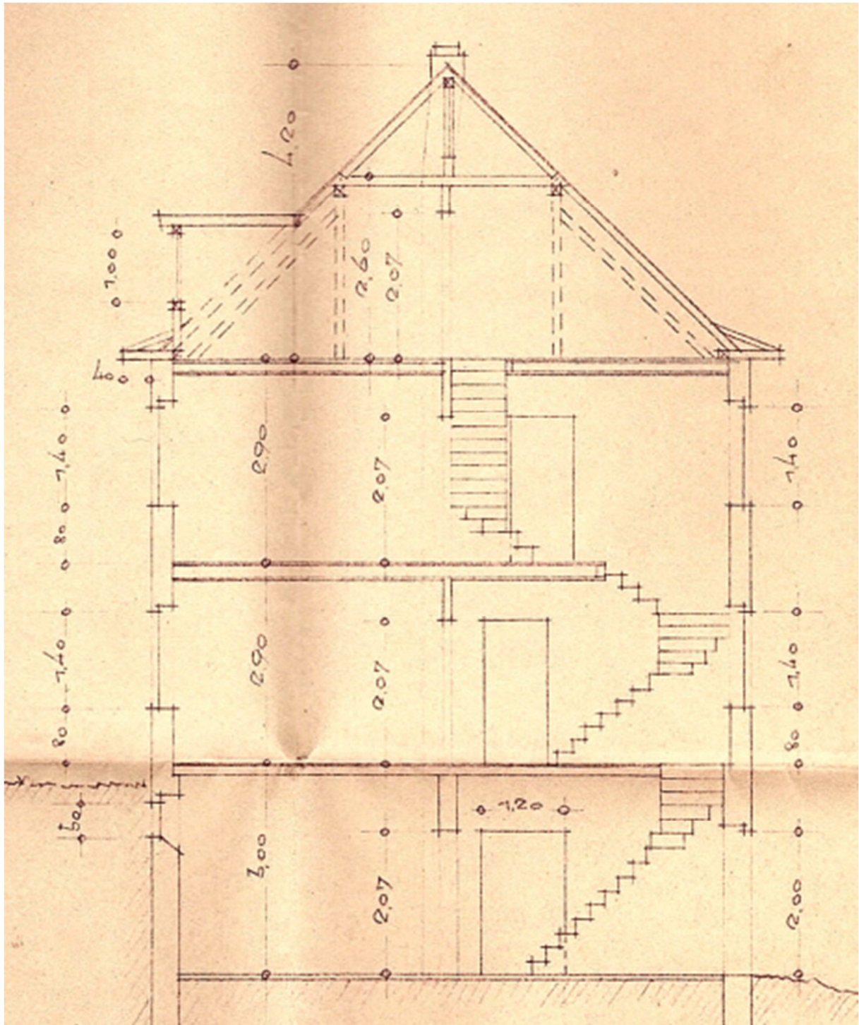
Haus-Querschnitt
