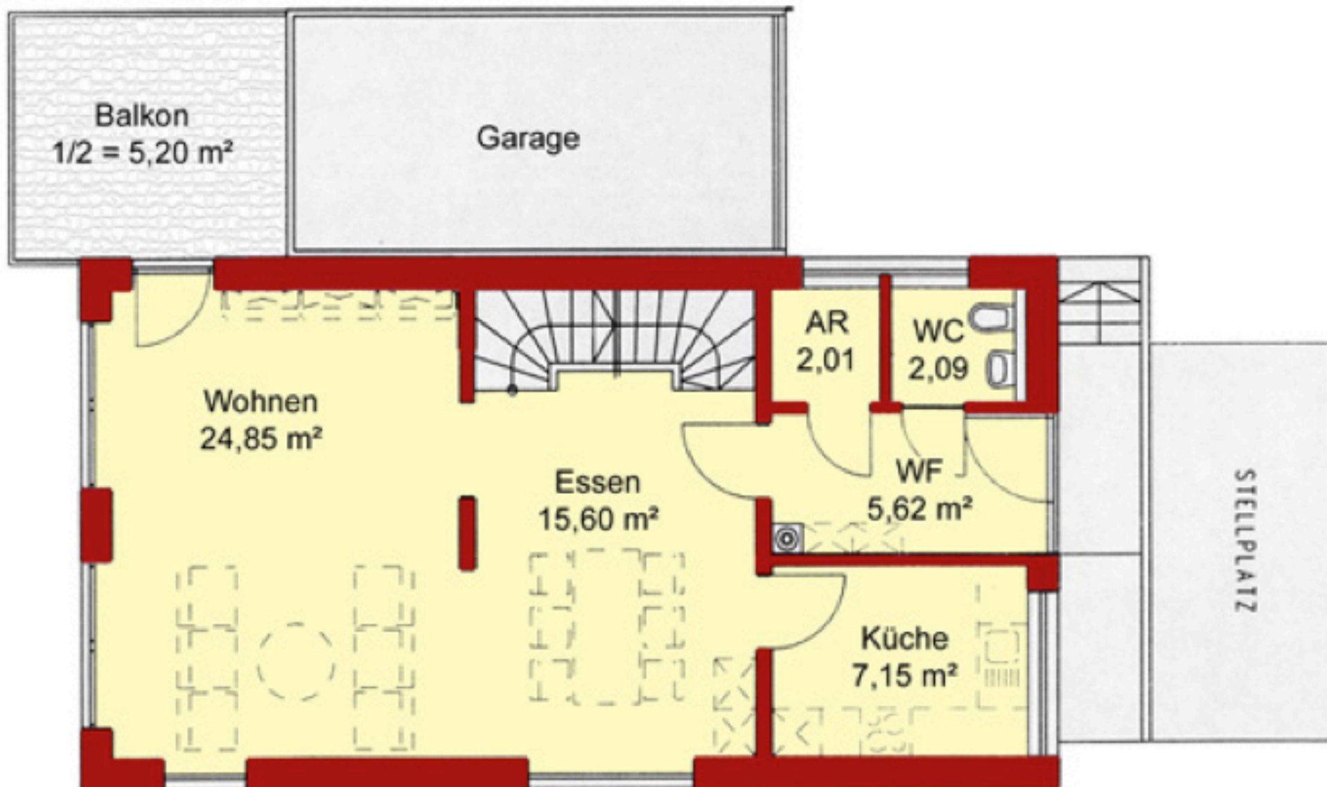
Erdgeschoss (Kein Maßstab)
