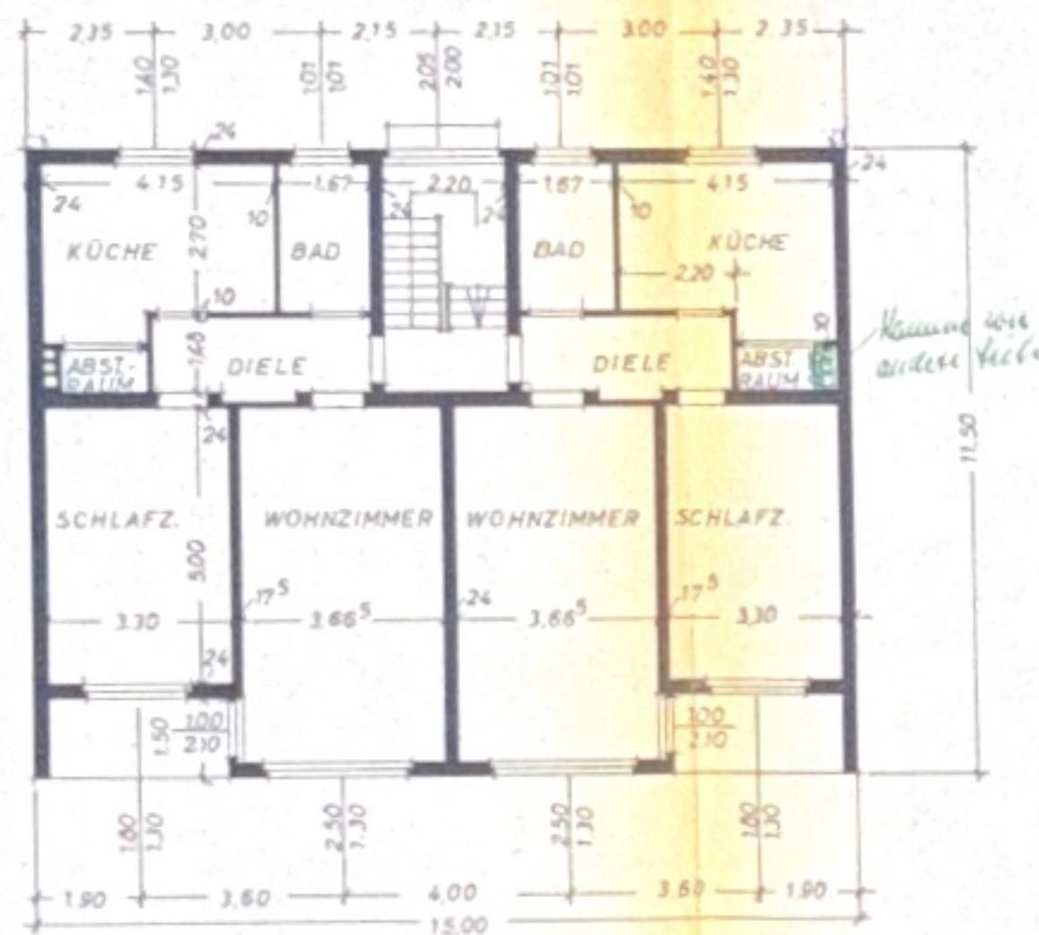
ERD- u. OBERGESCHOSS
