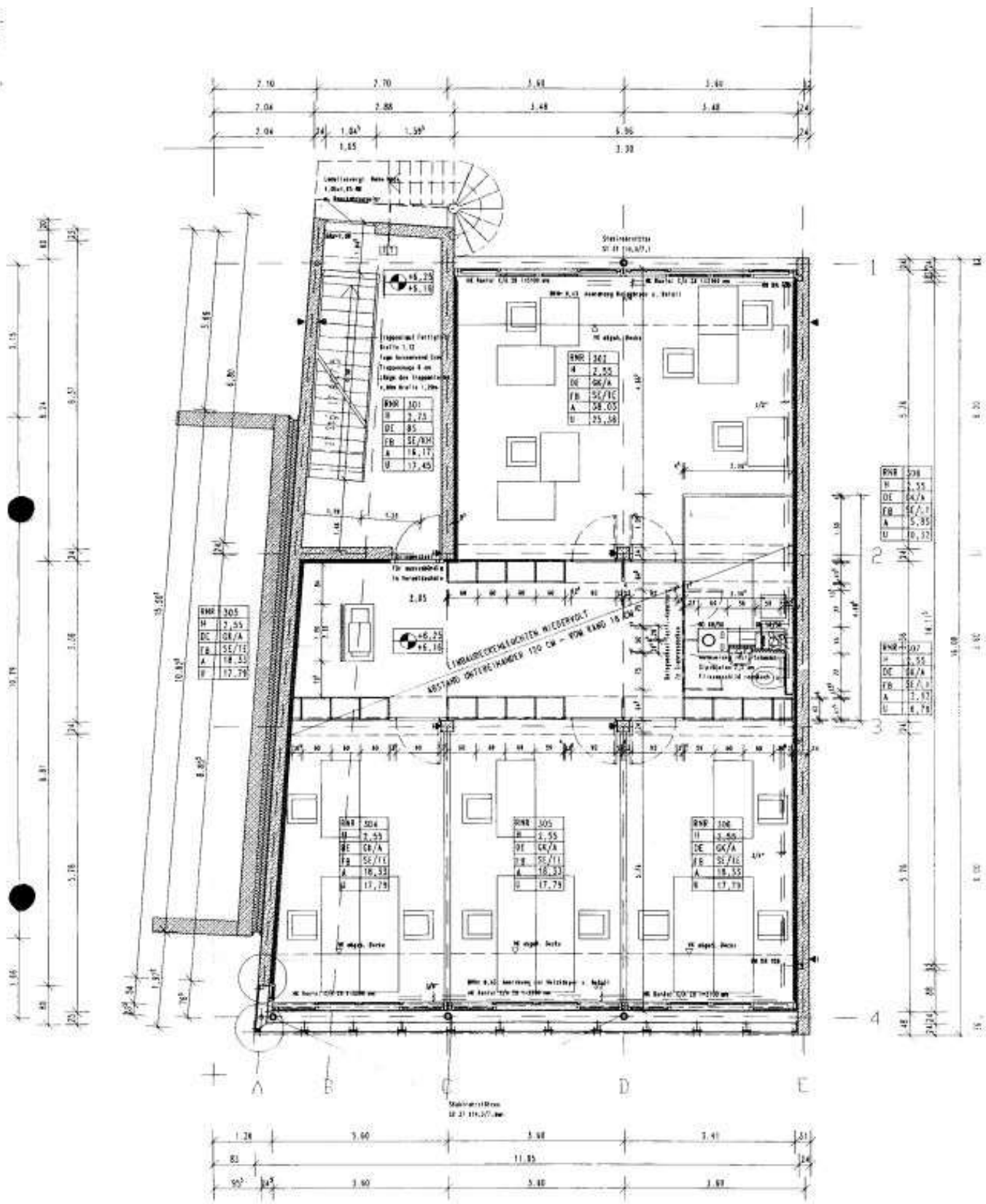
Grundriß 2. OG M. 1 : 100
