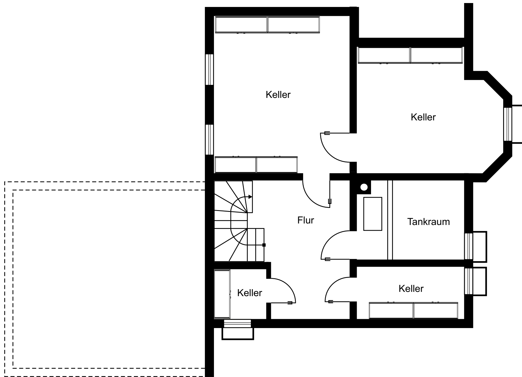
Kellergeschoss
