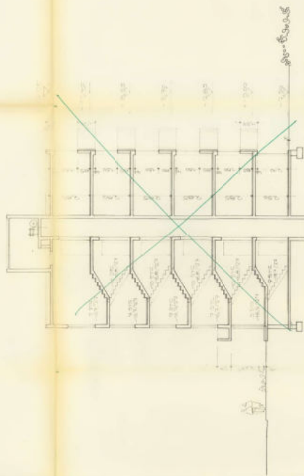
SCHNITT DURCH DEN ZWISCHENGANG ZW. 1. u. 2. ST.
