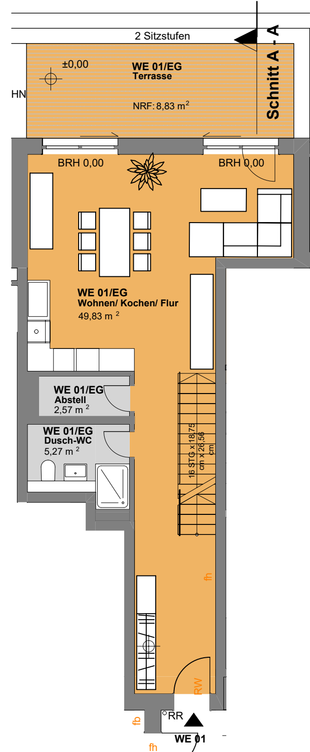
Wohnung 01 - Erdgeschoss
