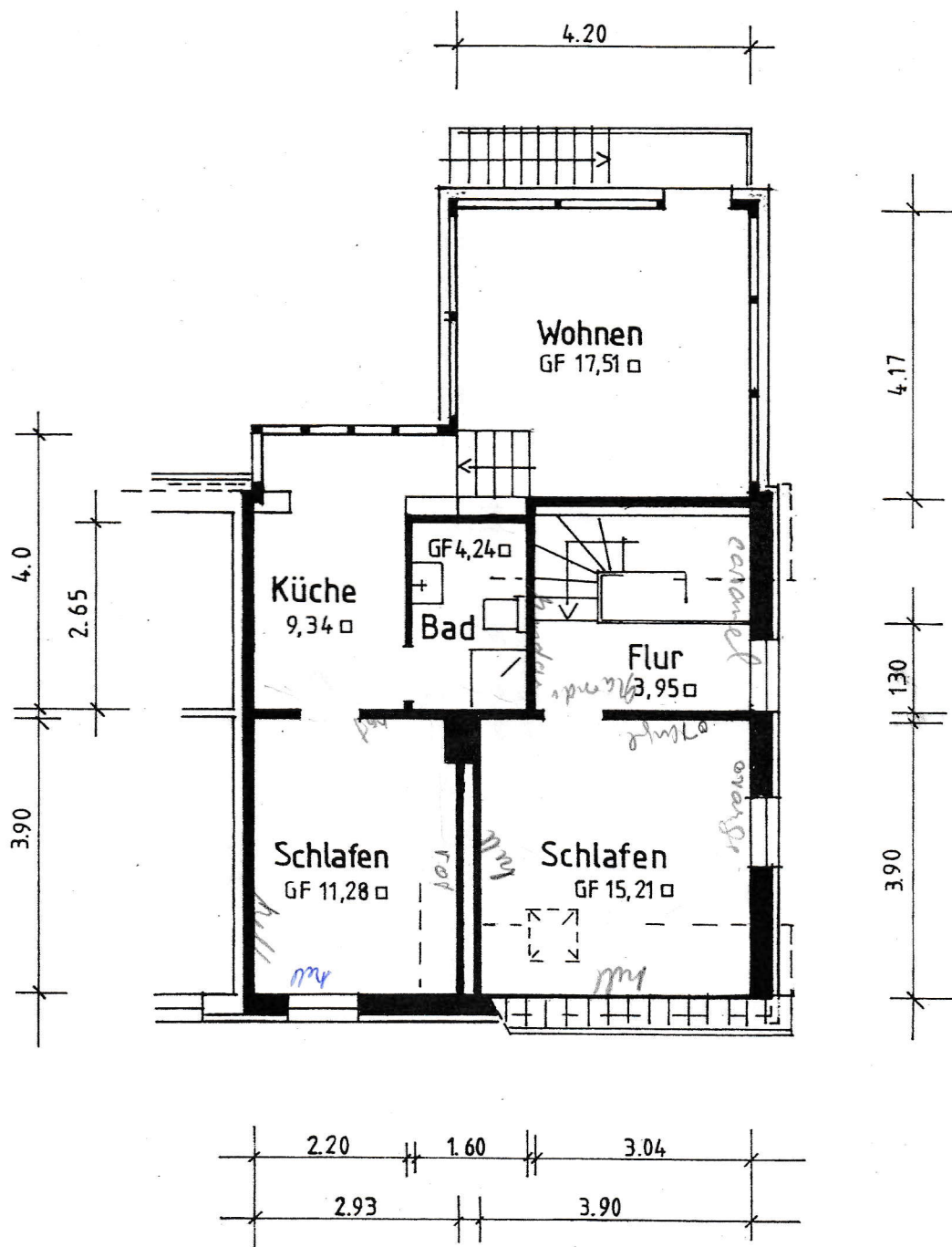
OBERGESCHOSS M.1:100
