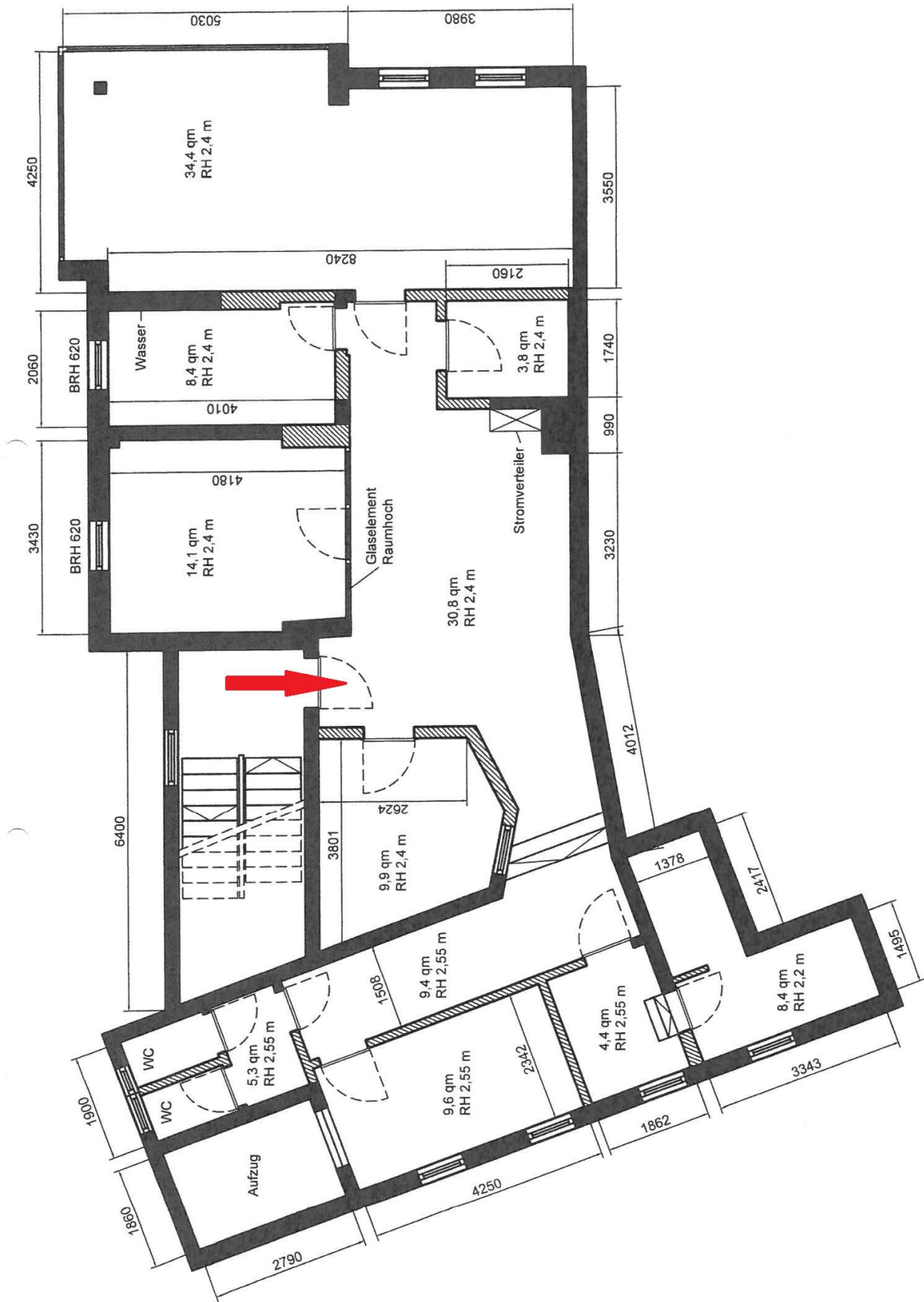
Grundriss Bürofläche (nicht maßstabsgetreu)
