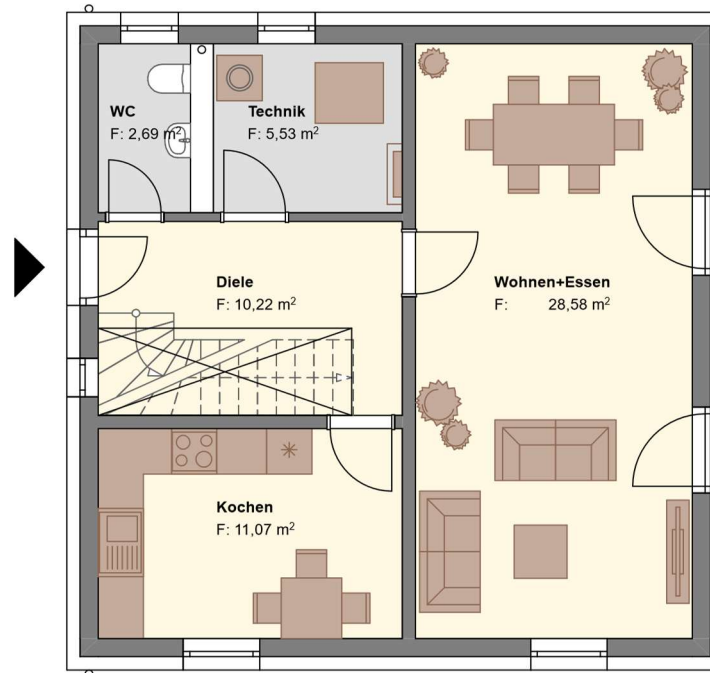
Erdgeschoss family 112 grün
