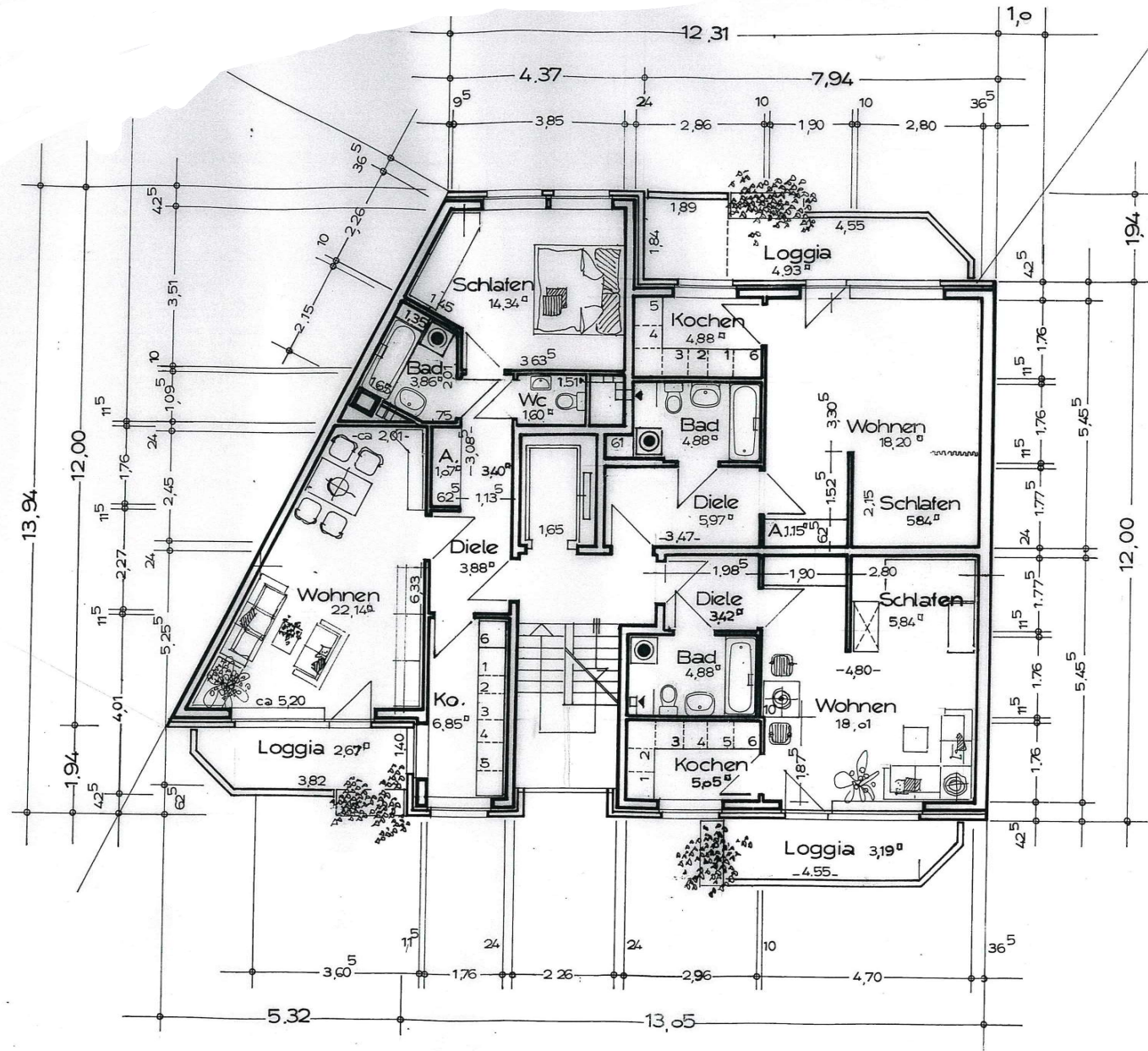
Grundriss 5. + 6. OG
