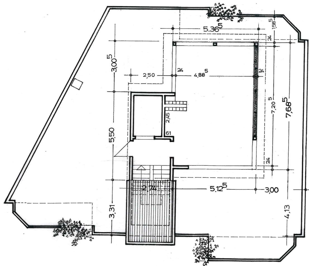
Grundriss Staffelgeschoss
