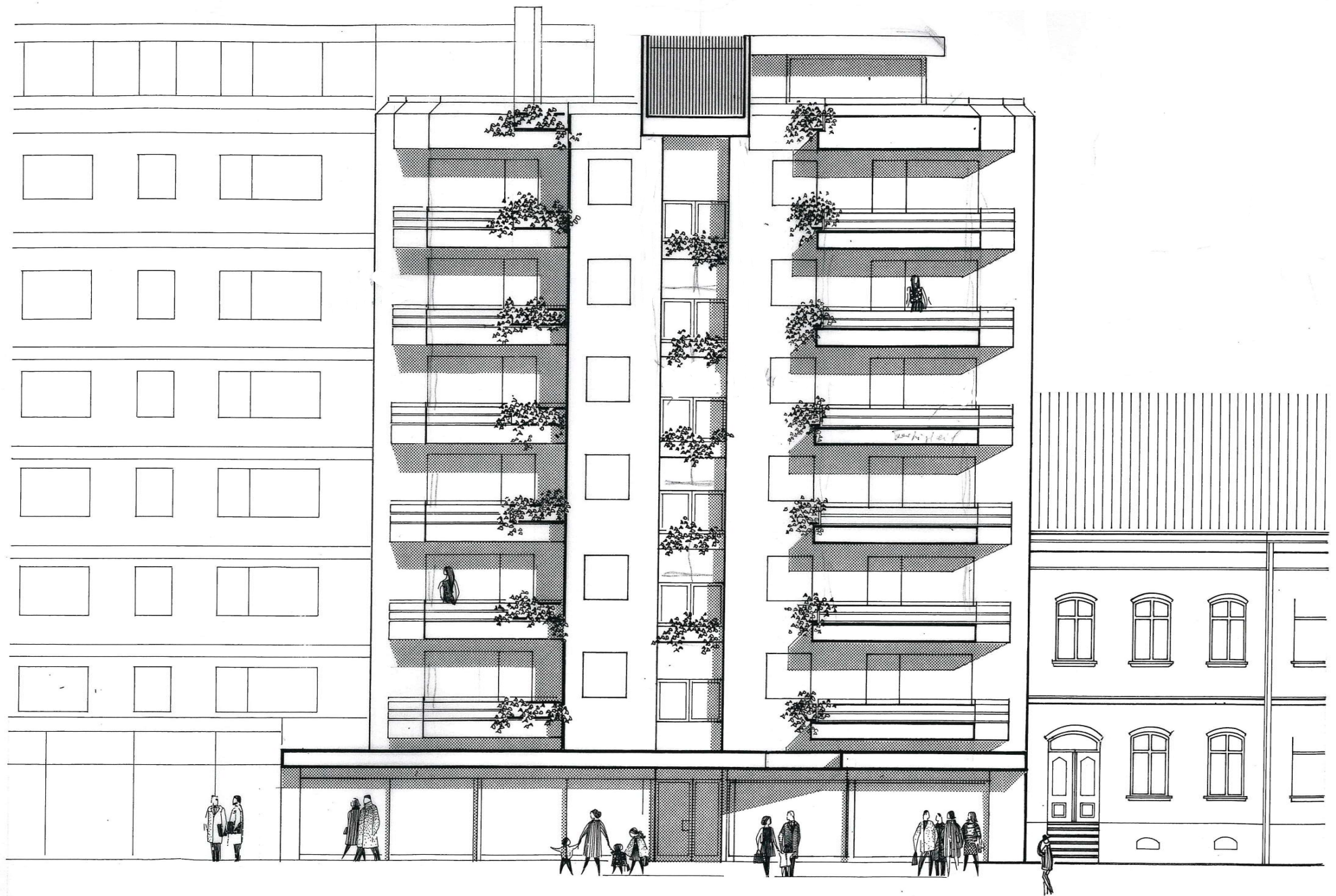
Strassenansicht
