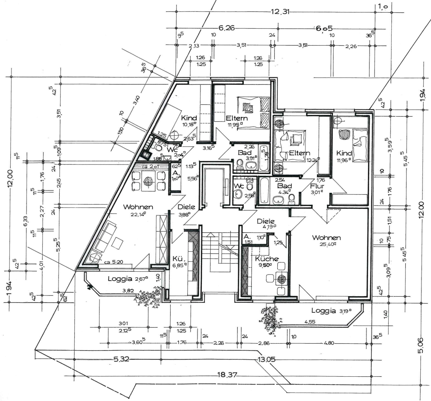
Grundriss 1.- 4. OG
