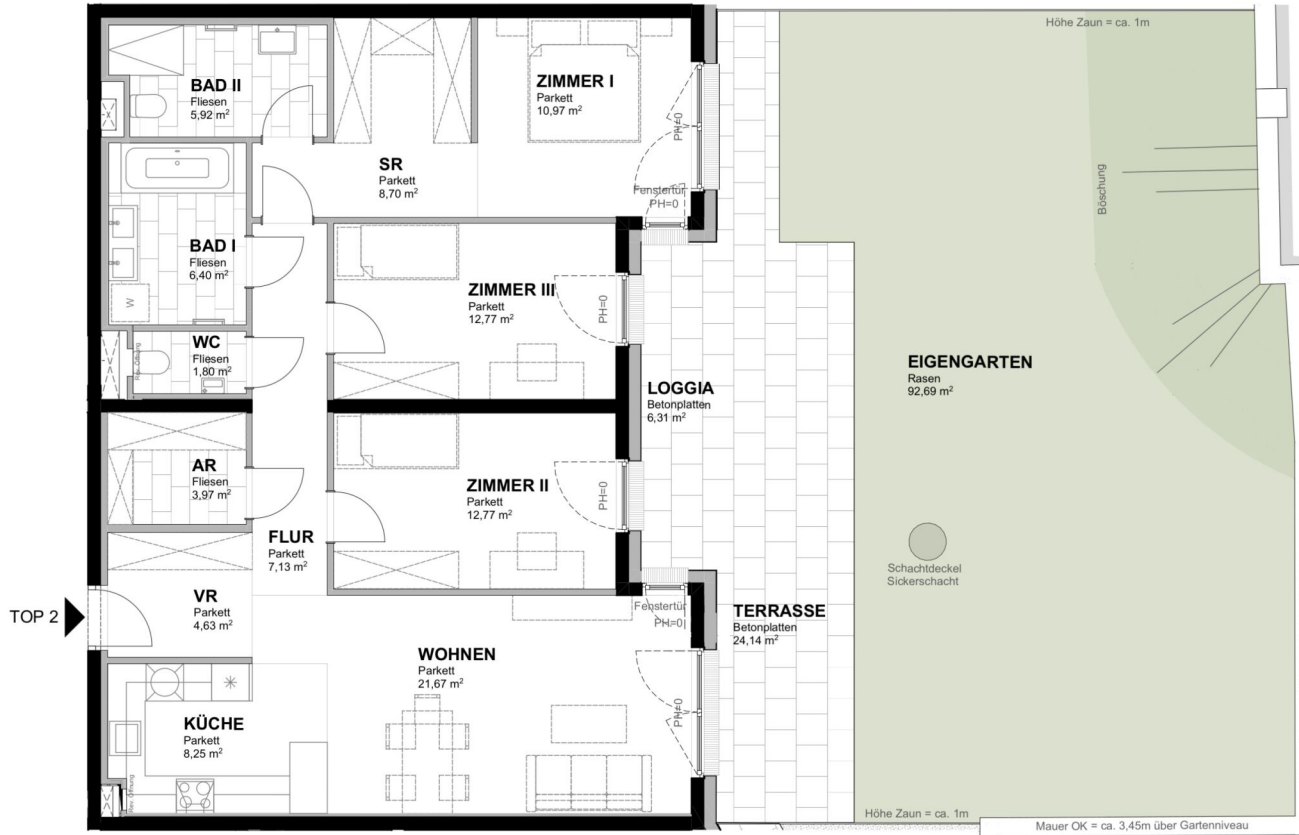
Übersichtsplan Erdgeschoss
