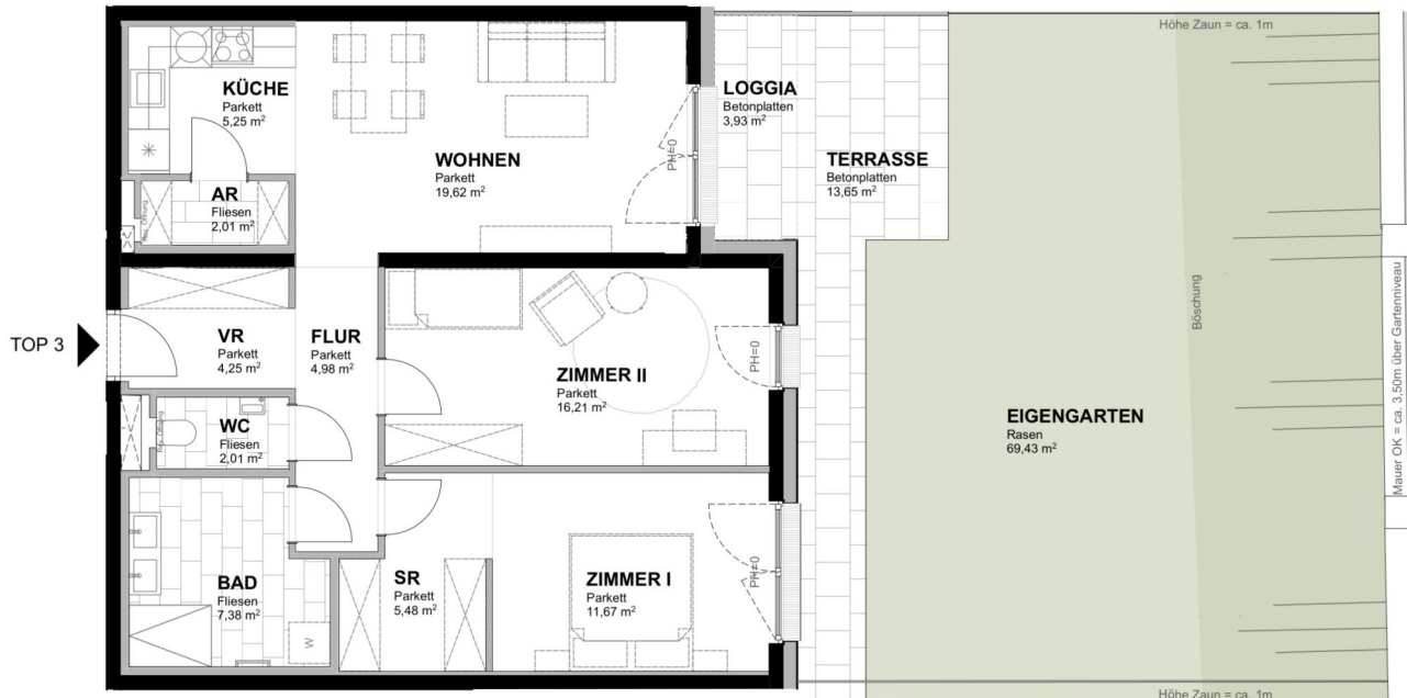
Übersichtsplan Erdgeschoss
