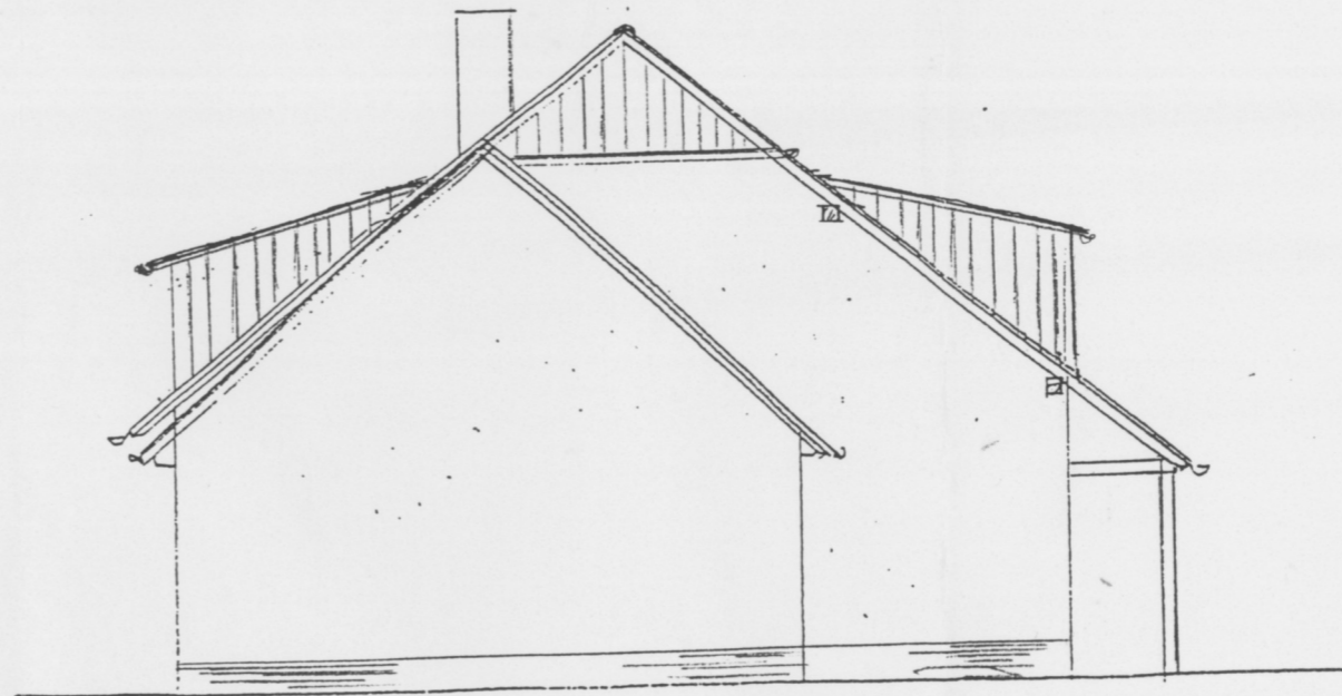
ANSICHT - WEST
