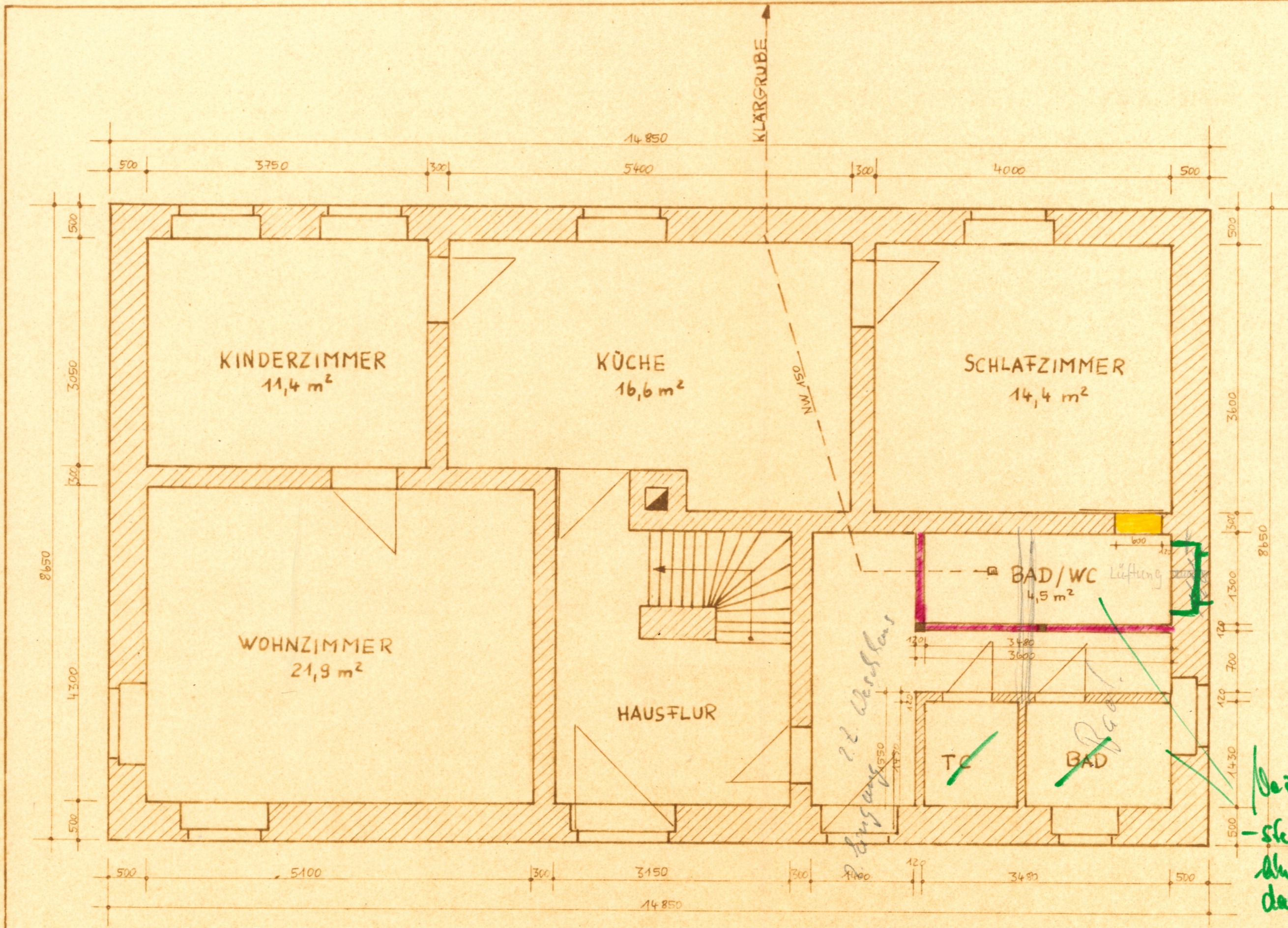
GRUNDRISS ERDGESCHOSS M 1:50
