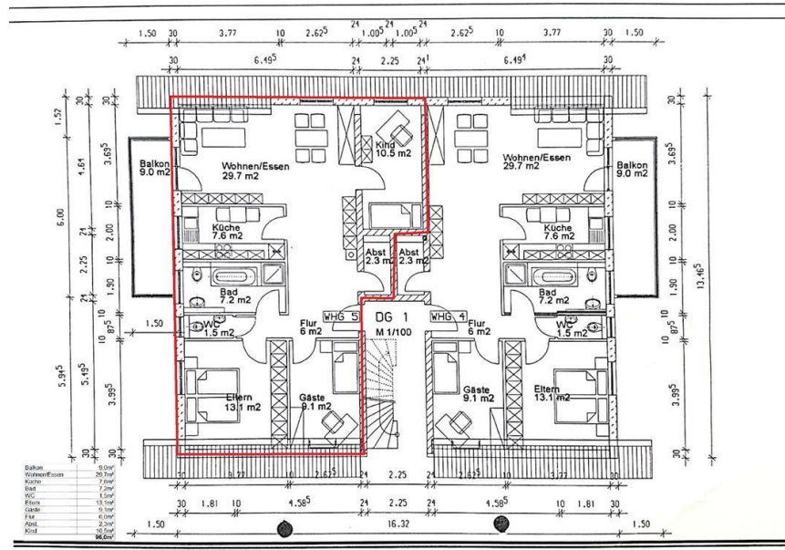
Grundrisse (Einzeichnung)
