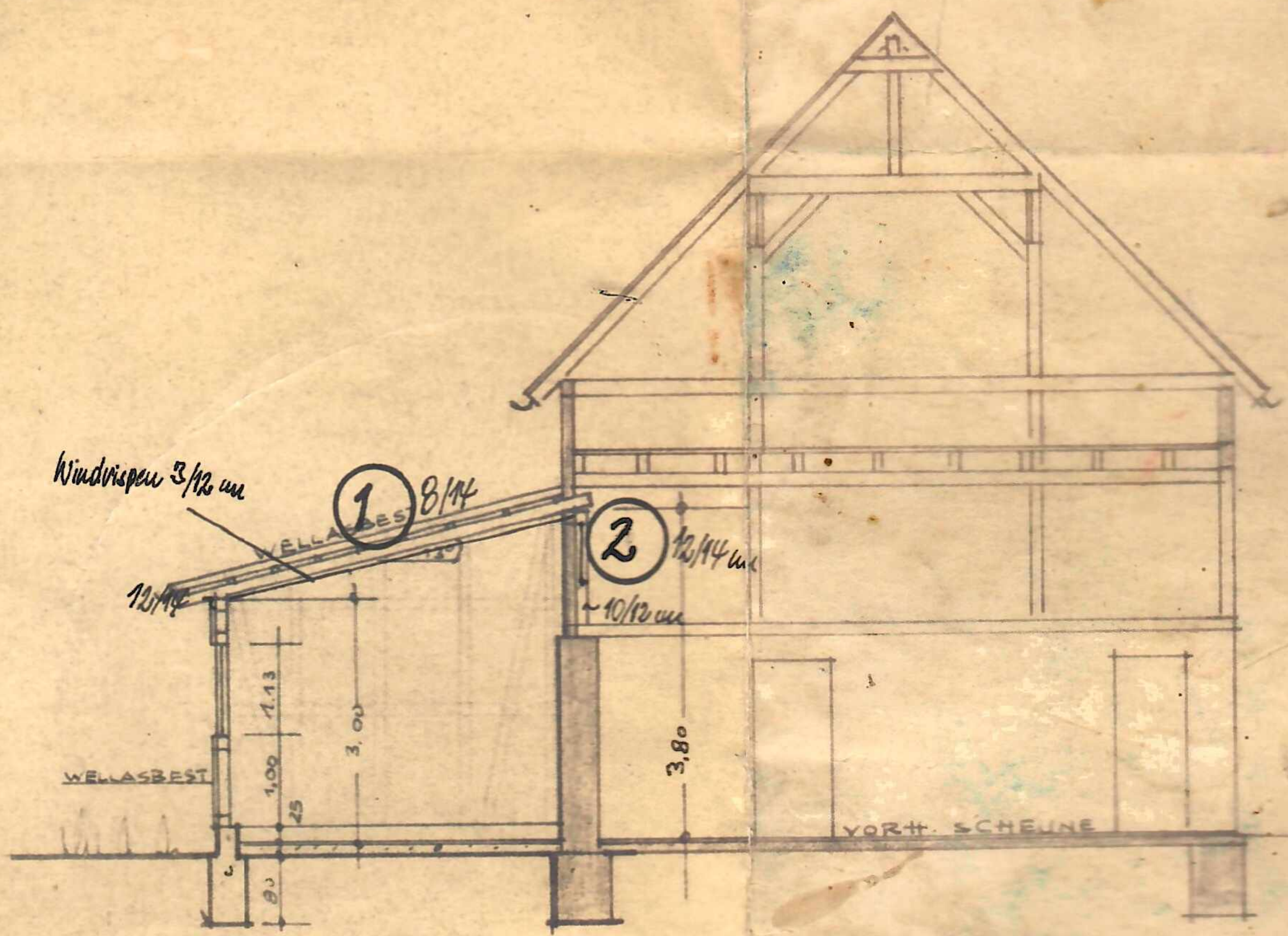
SCHNITT
