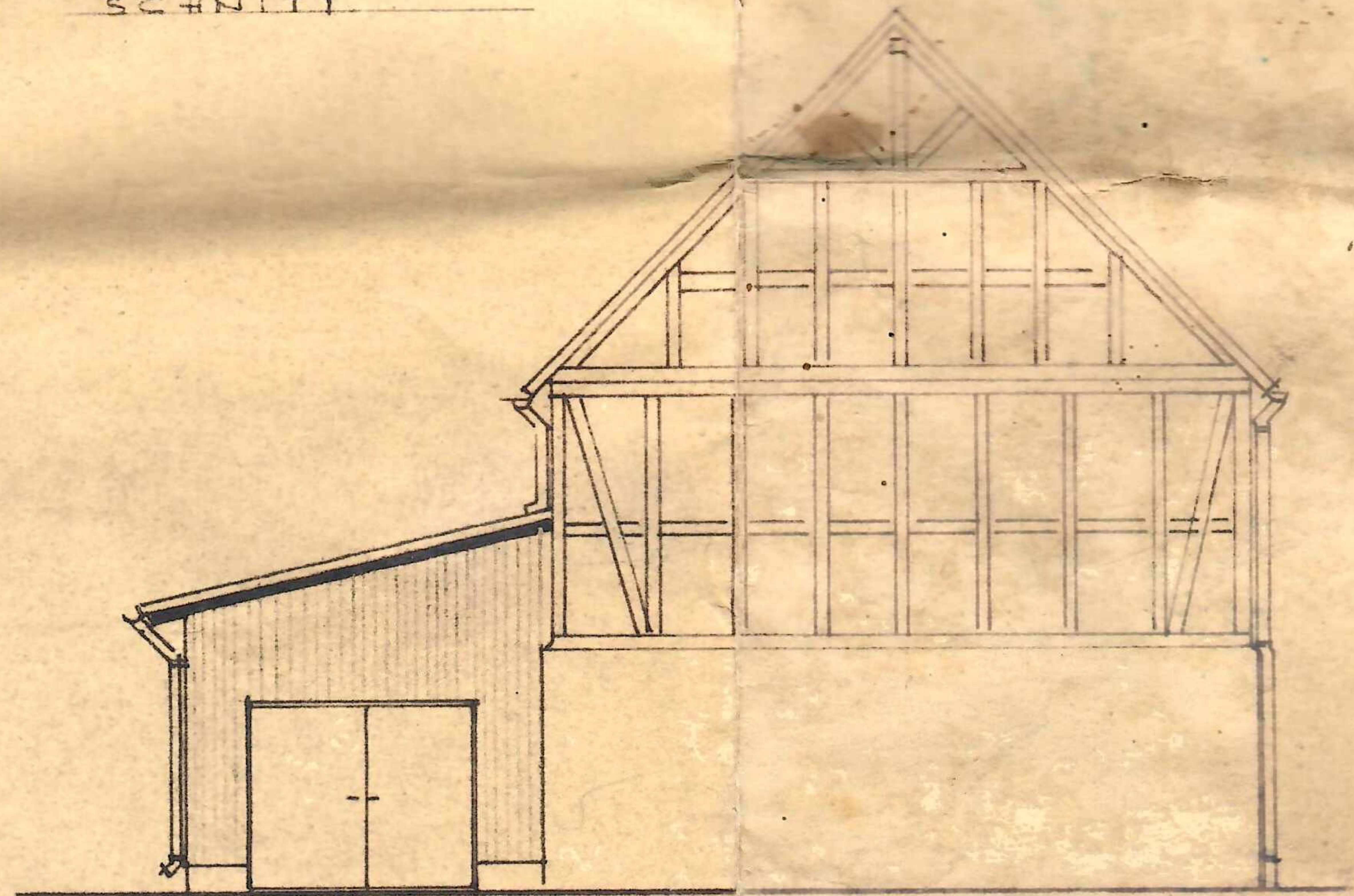
SCHNITT
