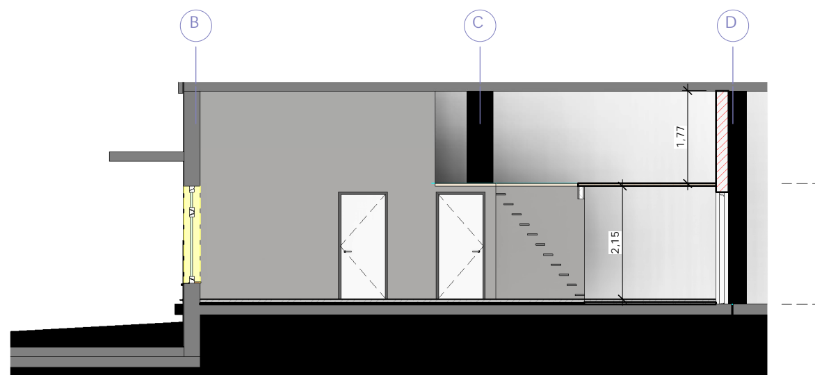
Systemschnitt "Längs"
