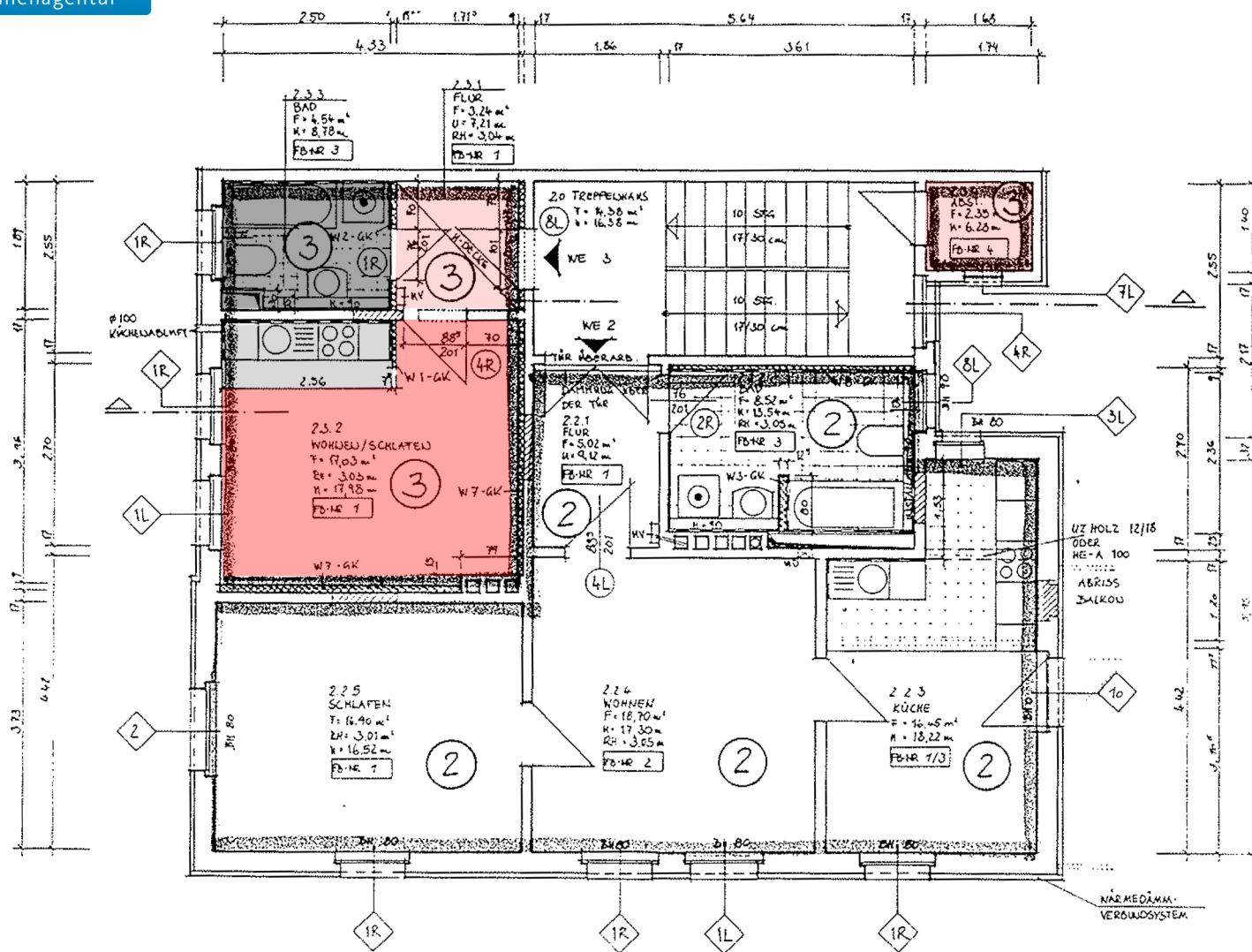
GRUNDRISS - Bockstraße 3 in 99423 Weimar 1 Zimmer-Küchenzeile auf 27,16qm im 1.OG
