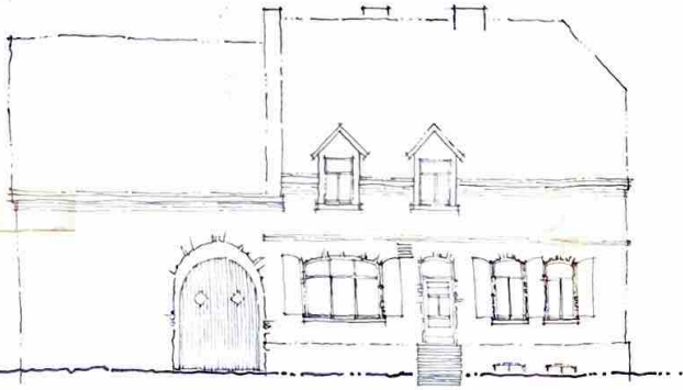
VORDERSEITE SÜDOST
