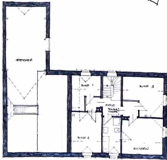
OBERGESCHOSS
