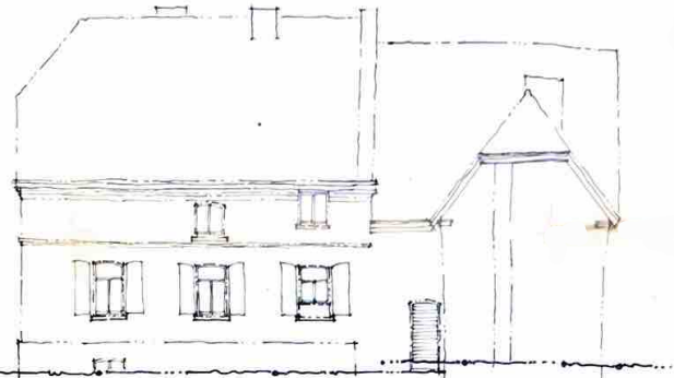
HOFSEITE NORDWEST
