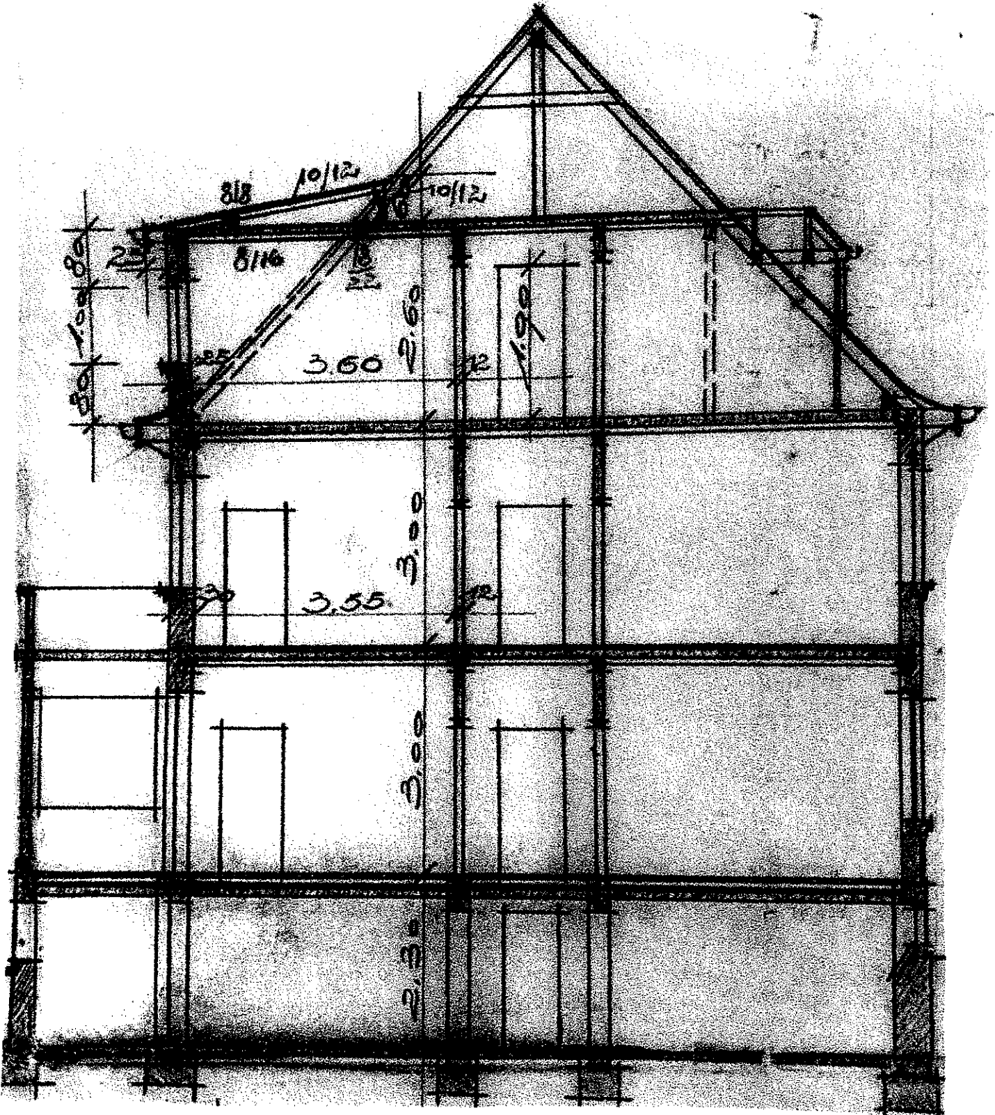
Schnitt
